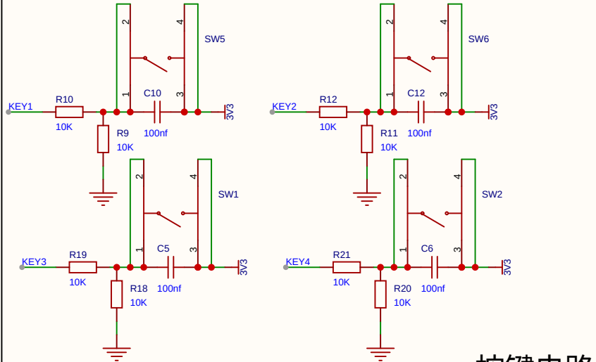
按键电路
