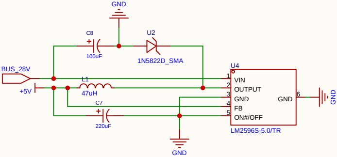
28V转5V电路
