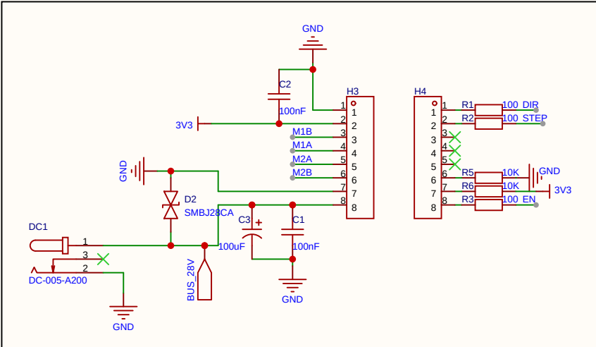
驱动输入电路
