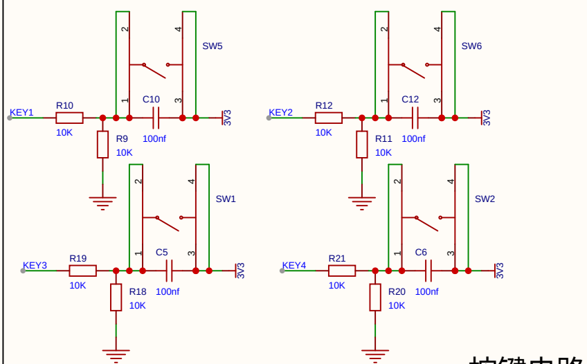
按键电路
