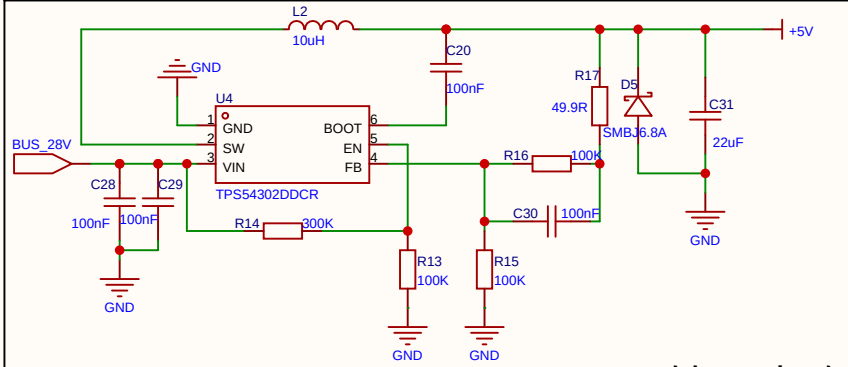
28V转5V电路
