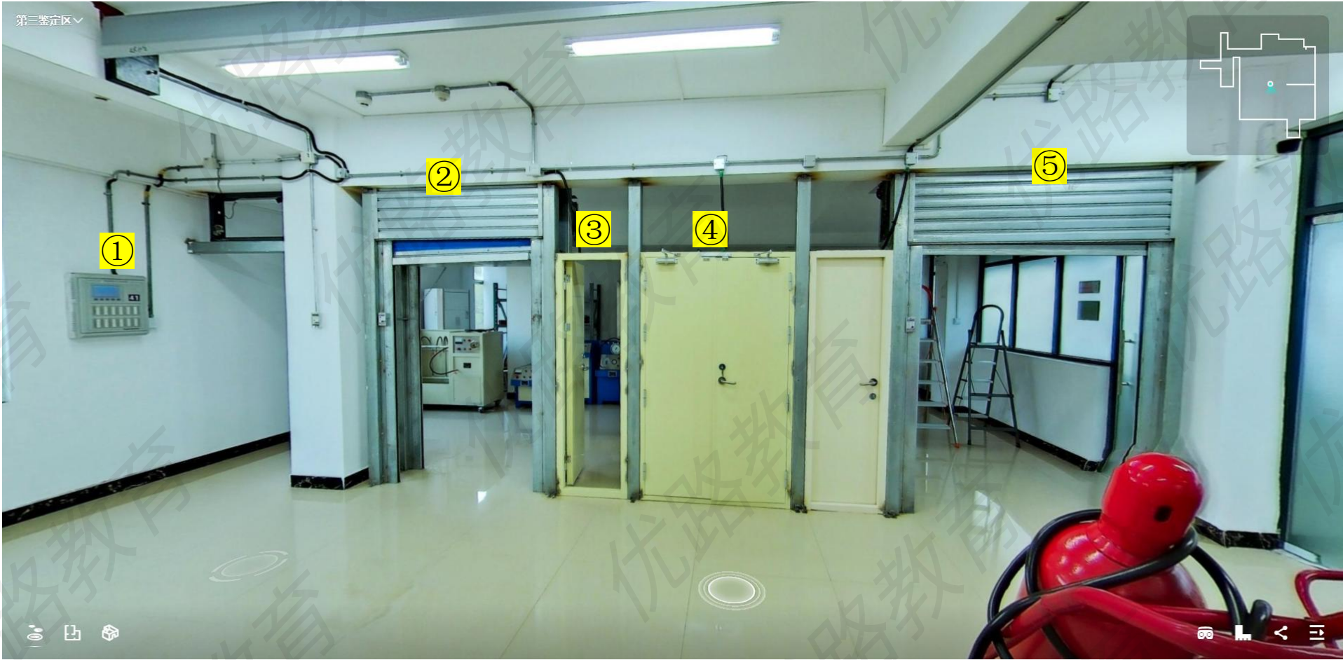
①防火门监控器②无机布防火卷帘③常开防火门④常闭防火门⑤钢制防火卷帘
