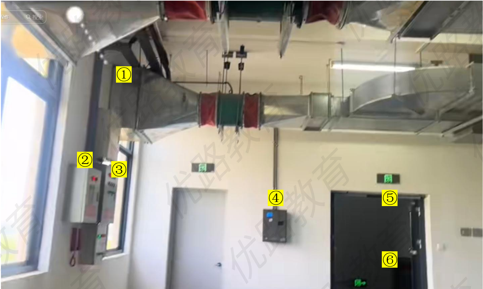
①排烟系统②双电源箱③排烟风机控制柜④防火门监控器【松江】⑤防火门⑥送风口 ★ 从防火门进去左转是防烟系统
