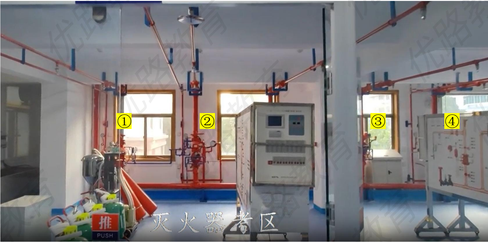
①干式系统②预作用系统③雨淋系统④湿式系统 ☆ 进门从左至右
