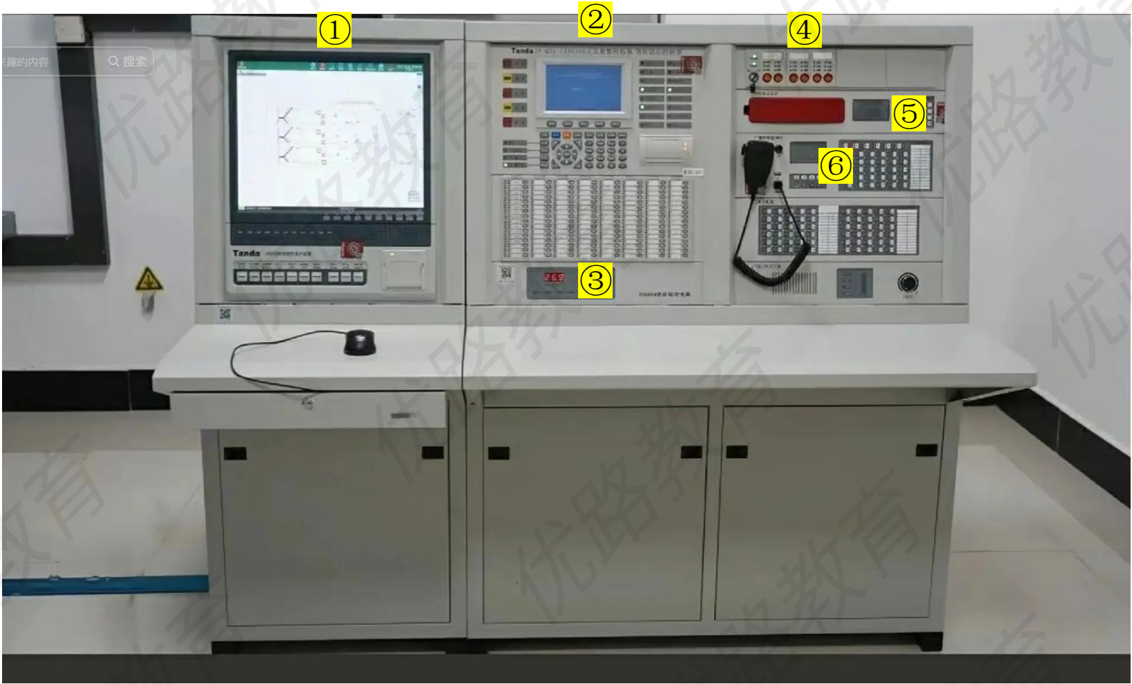
①消防控制室图形显示装置②集中火灾报警控制器③总线控制盘④多线控制盘⑤消防电话总机⑥消防应急广播
