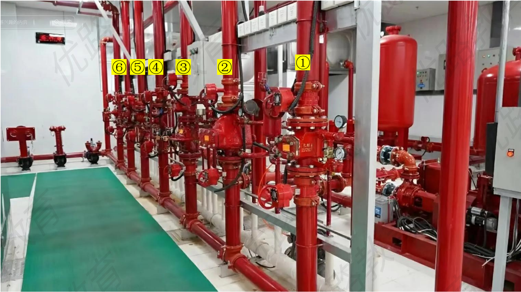
①湿式系统②干式系统③预作用系统
