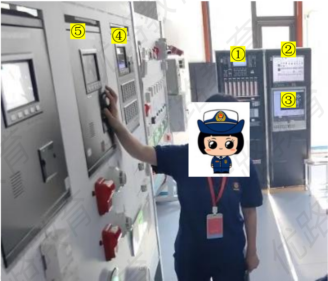
①集中火灾报警控制器②消防控制室图形显示装置 ③应急照明控制器④防火门监控器⑤可燃气体报警控制器 ★ 主机品牌：泰和安3016C（24年8月新增机型）
