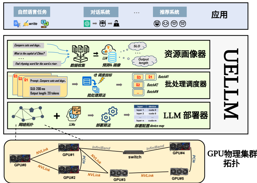
图 3-1 UELLM 系统整体架构图 [13]
