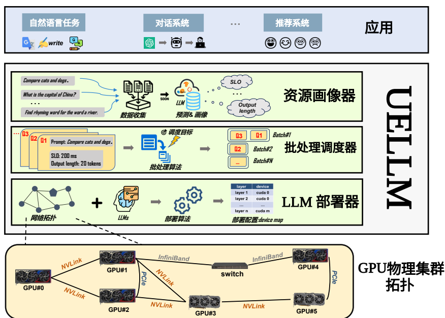
图 3-1 UELLM 系统整体架构图 [12]
