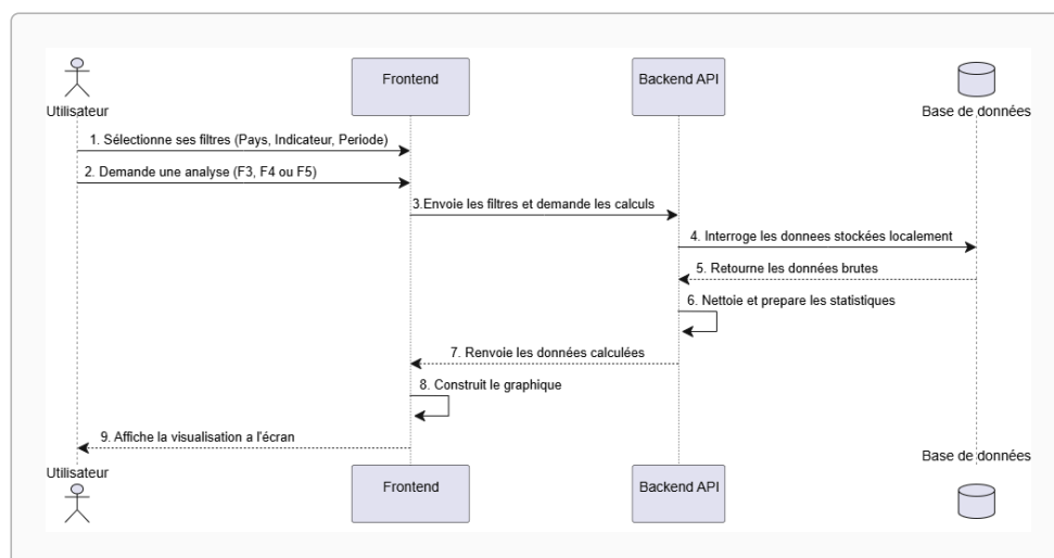
Fig. 3 — Diagramme de séquence - fonctionnalité
