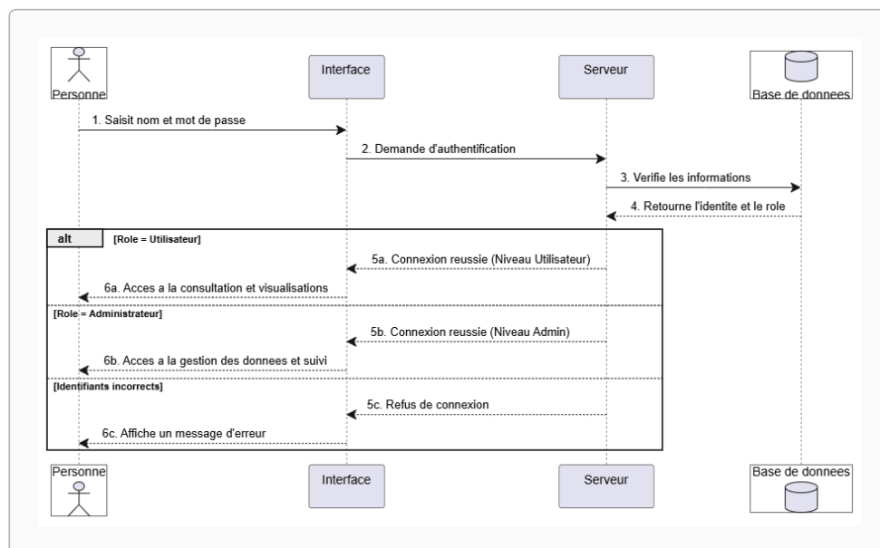
Fig. 4 — Diagramme de séquence - authentification
