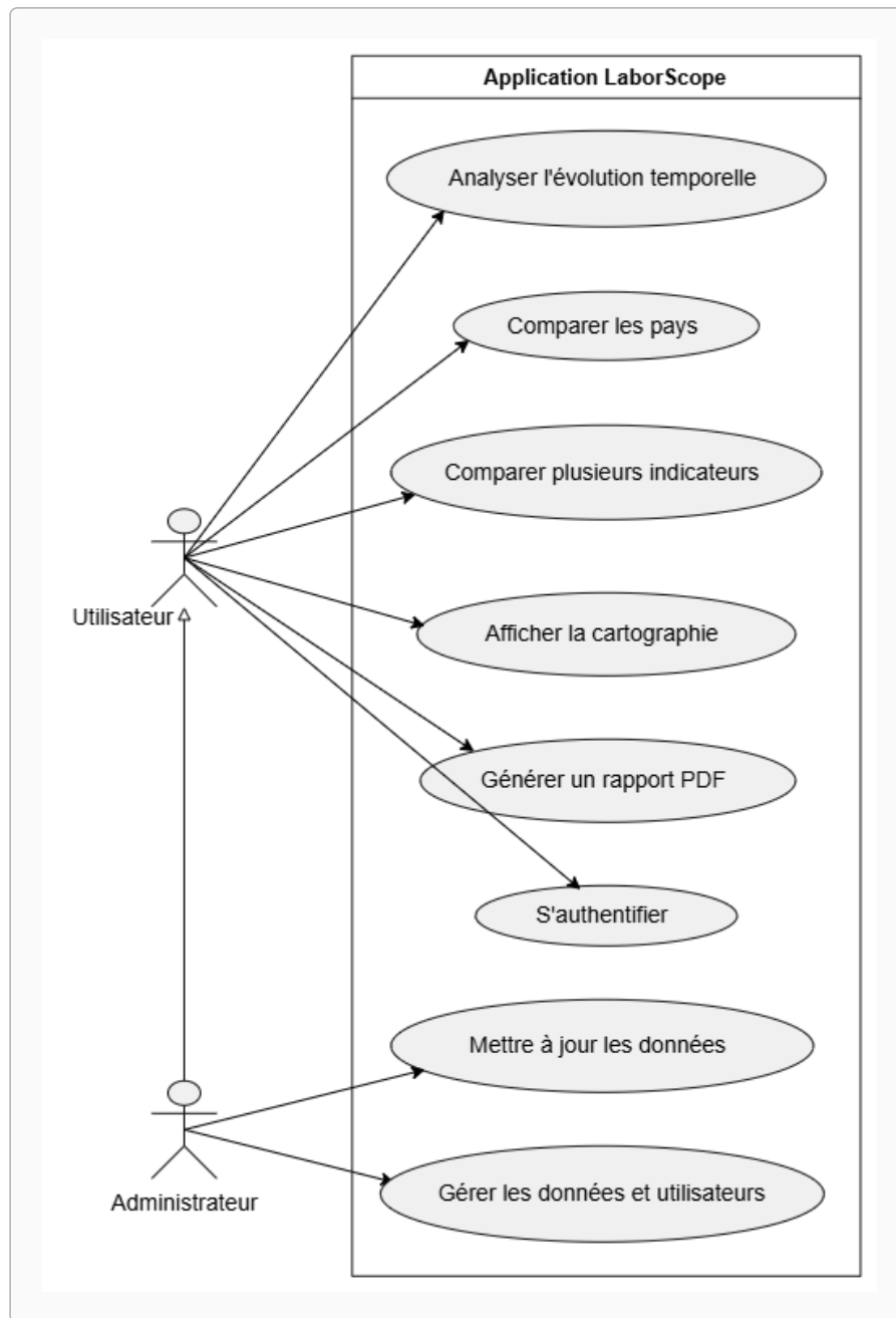
Fig. 1 — Diagramme de cas d'utilisation
