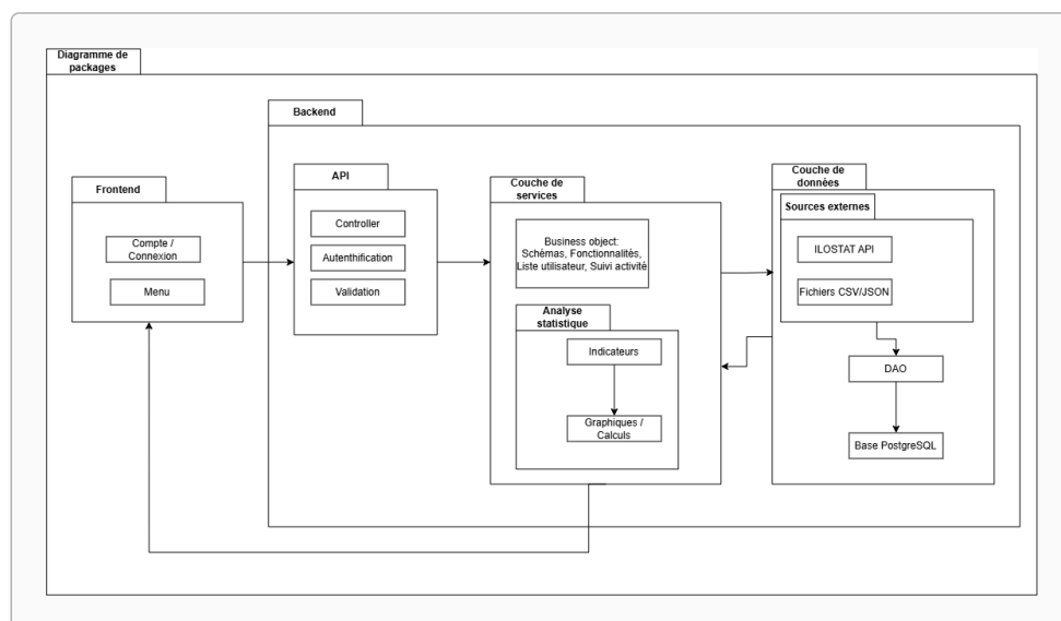
Fig. 5 — Diagramme de packages
