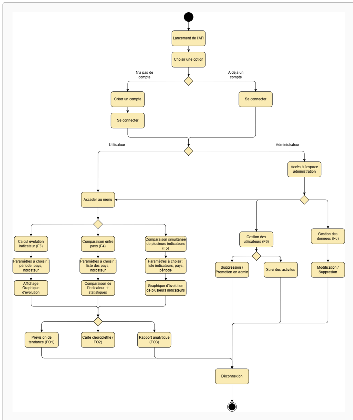
Fig. 2 — Diagramme d'activité
