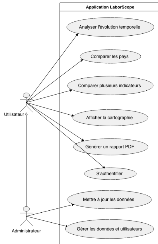
Figure 1. – Diagramme de cas d'utilisation
