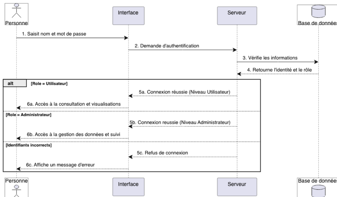
Figure 3. – Diagramme de séquence (authentification)
