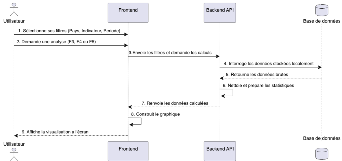
Figure 4. – Diagramme de séquence (données analytiques)
