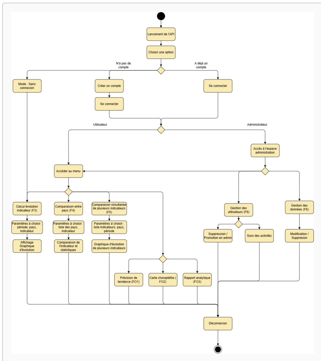
Fig. 2 – Diagramme d'activité
