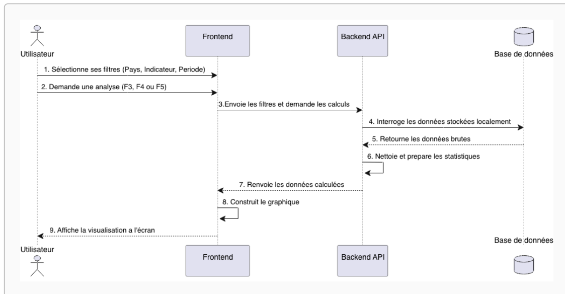
Fig. 7 — Diagramme de séquence - analyse
