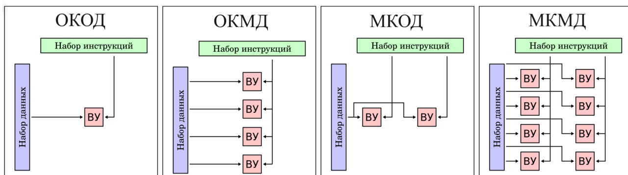
Рис. 15 — Все виды архитектур по таксономии Флинна
