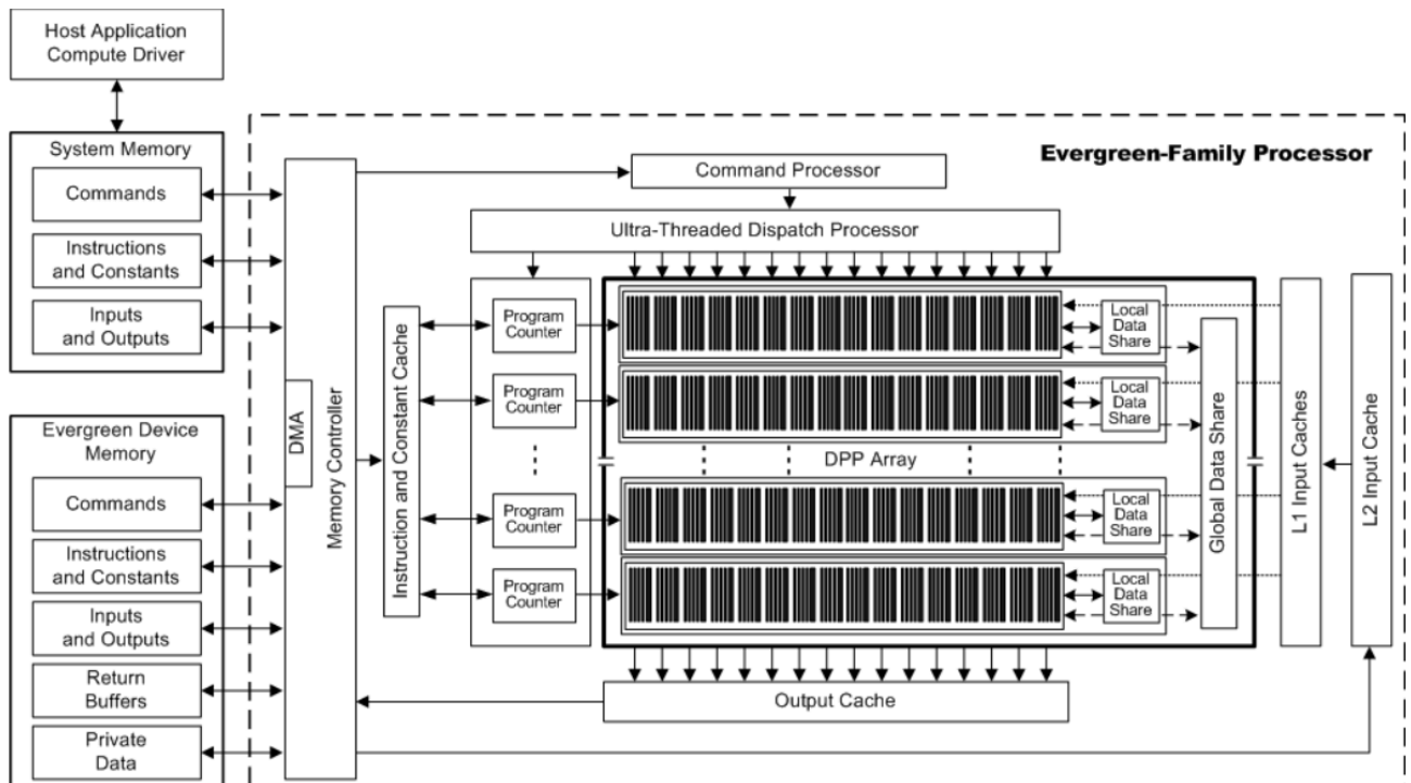
Рис. 9 — Графический процессор семейства Evergreen
