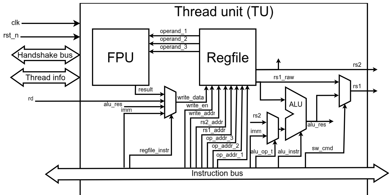
Рис. 19 — Упрощенная схема блока потока (Thread Unit)
