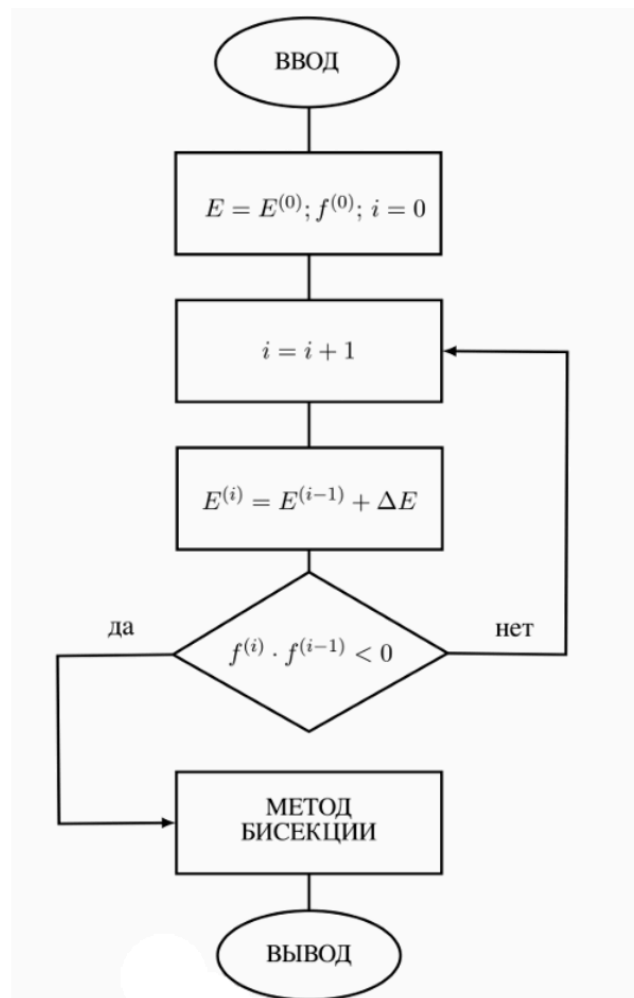
Рис. 3 — Блок-схема процедуры поиска собственного значения
