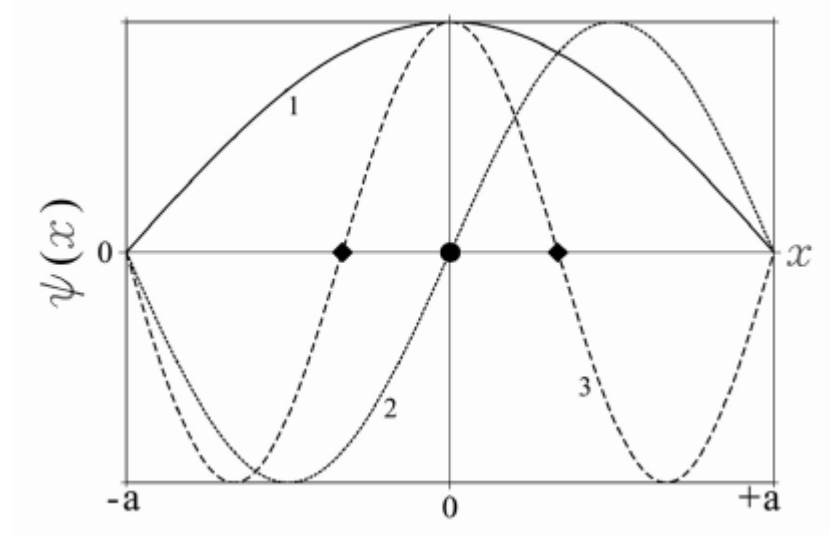
Рис. 2 — Прямоугольная потенциальная яма с бесконечными стенками: волновые функции \psi_1(x) , \psi_2(x) и \psi_3(x)
