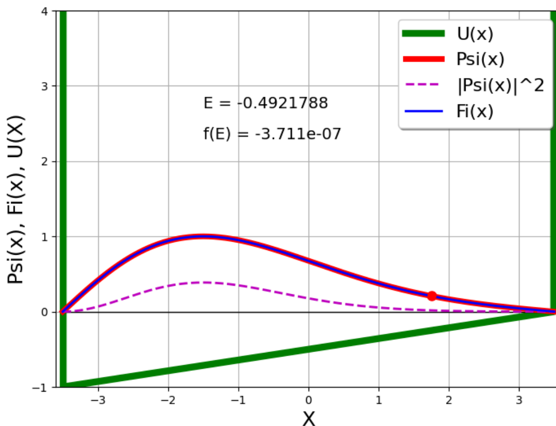
Рис. 4 — Волновая функция и плотность вероятности основного состояния
