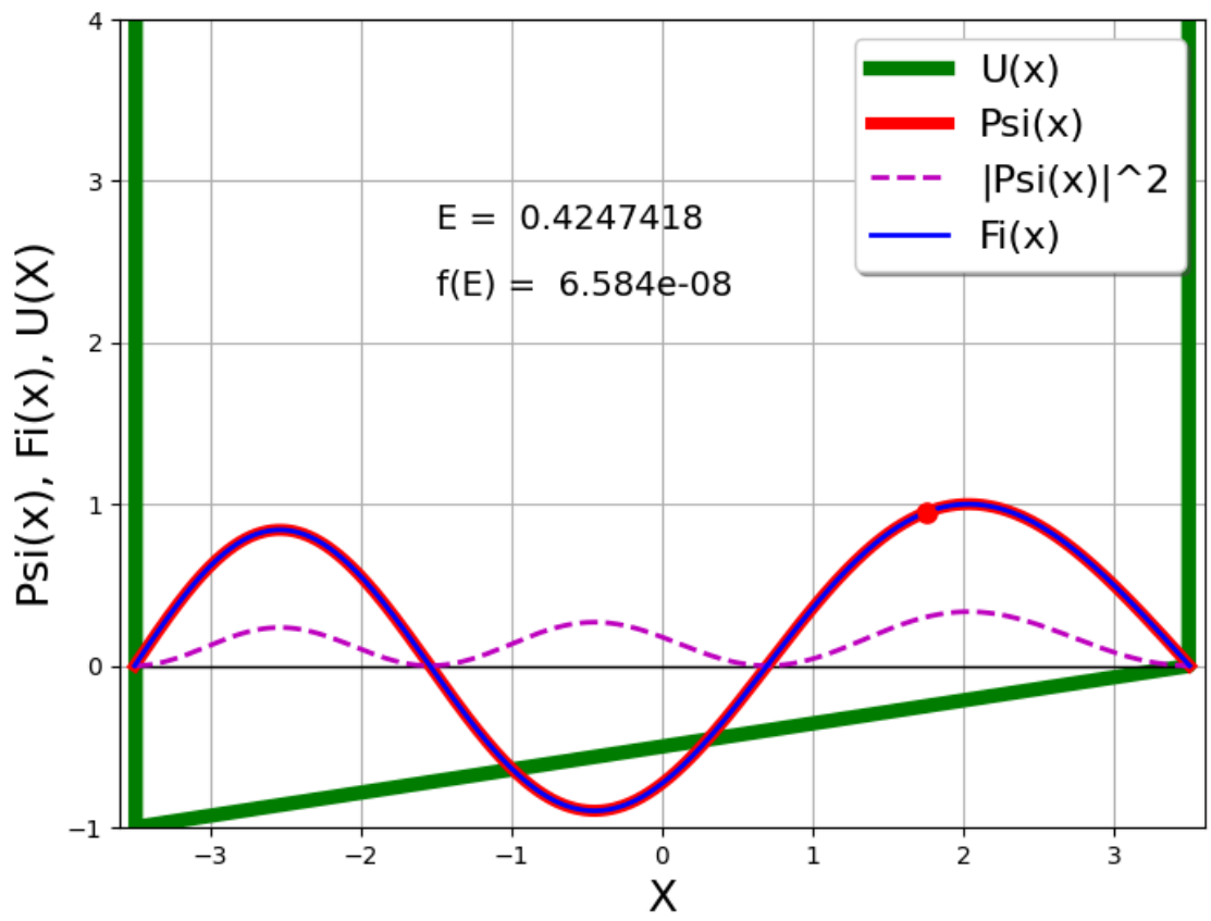
Рис. 5 — Волновая функция и плотность вероятности k = 2 возбужденного состояния
