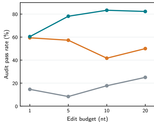
D SK-N-SH
