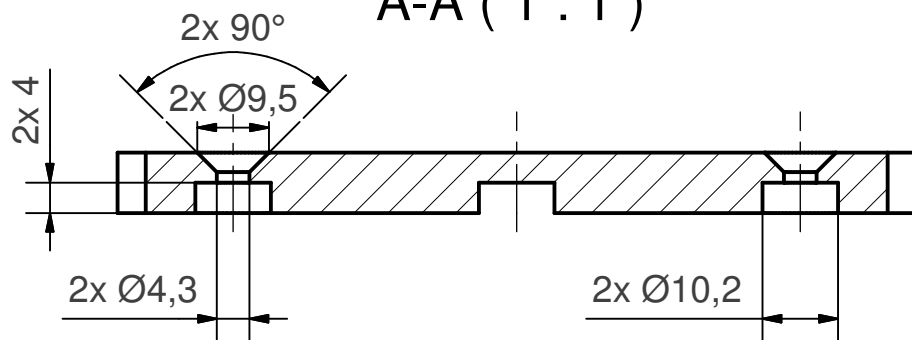
A-A ( 1 : 1 )
