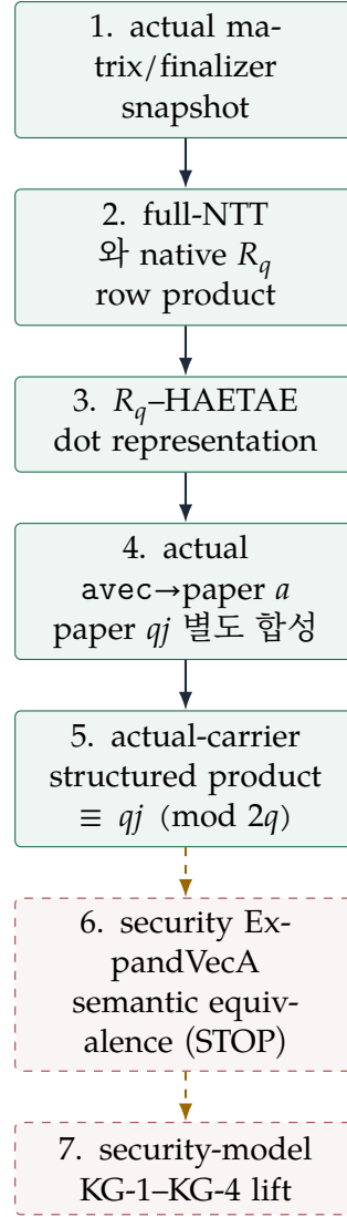
그림 4: post-freeze KeyGen의 현재 절단면. actual-carrier 전용 coefficient-product까지 달렸지만, generic security ExpandVecA/matrix_vec_mul 의미론에서 중단했다.
