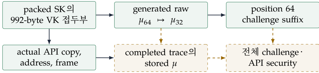
그림 2: key/transcript 진행선. 실선은 닫힌 정리(theorem), 점선은 열린 승격이다.
