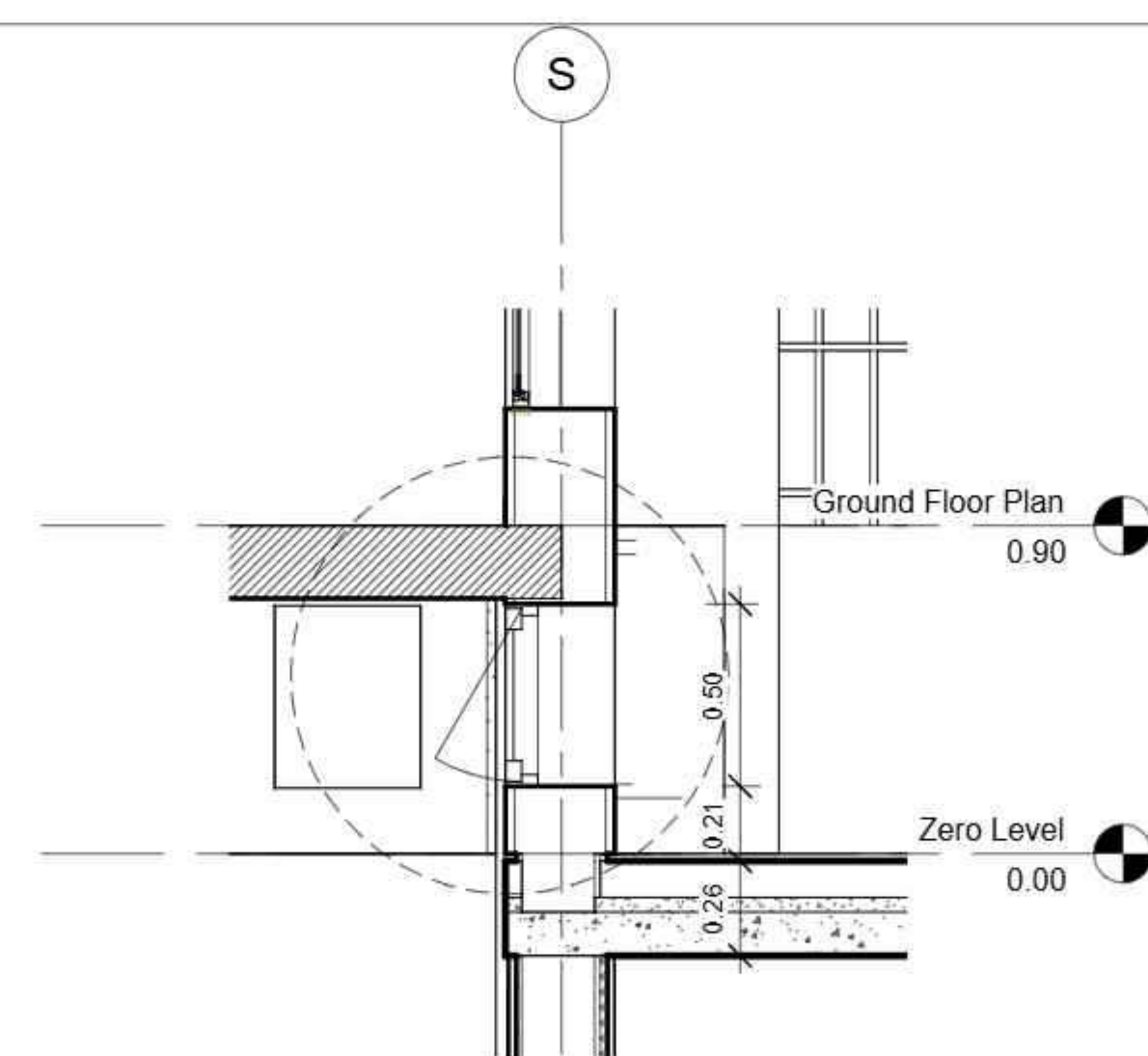
3 Basement Windows Details 1 : 20
