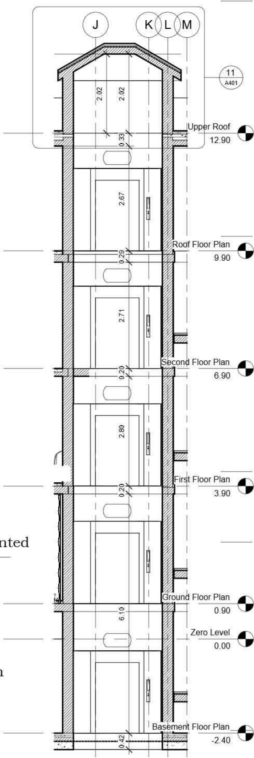
Elevator Section 1 : 50
