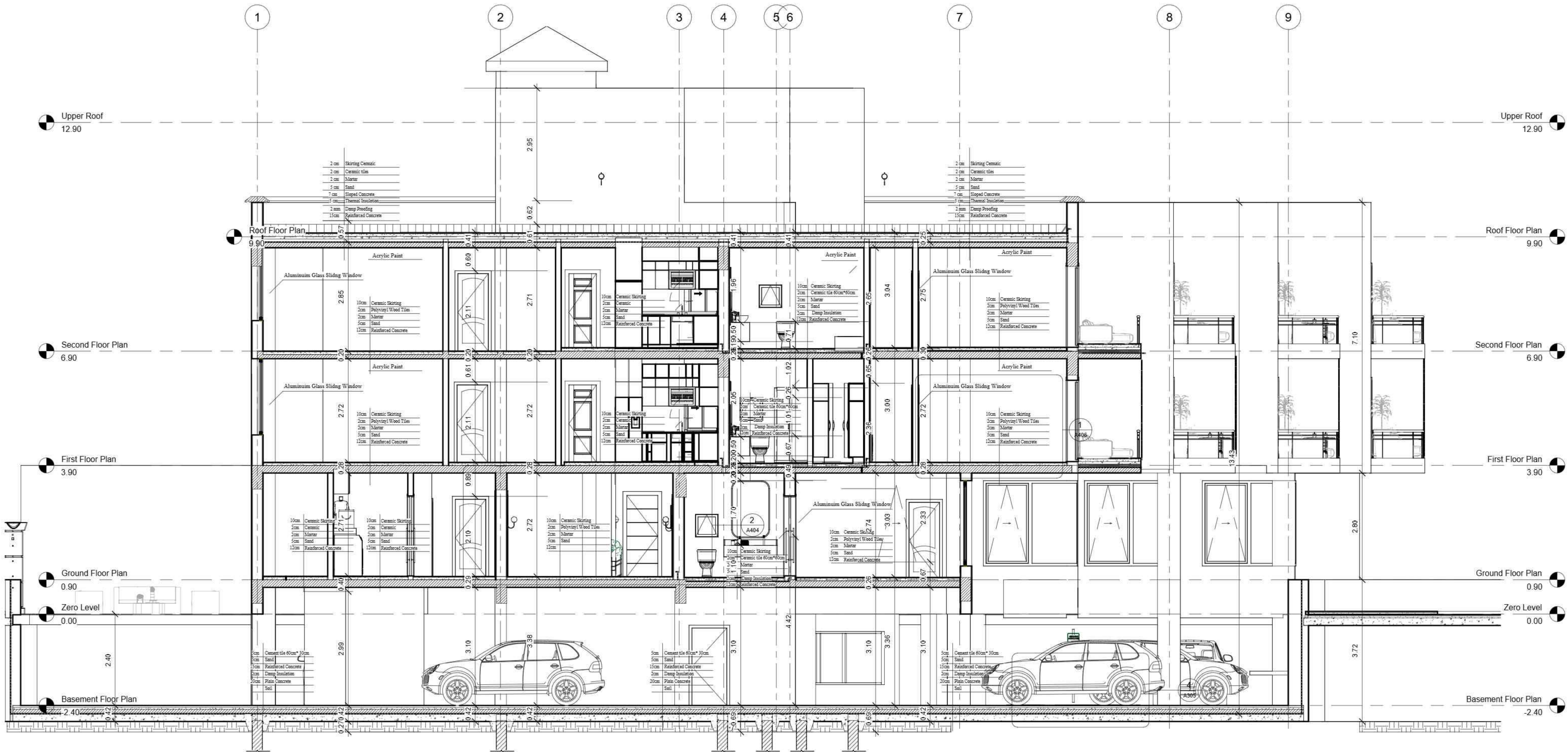
1 Side Section 1 : 50
