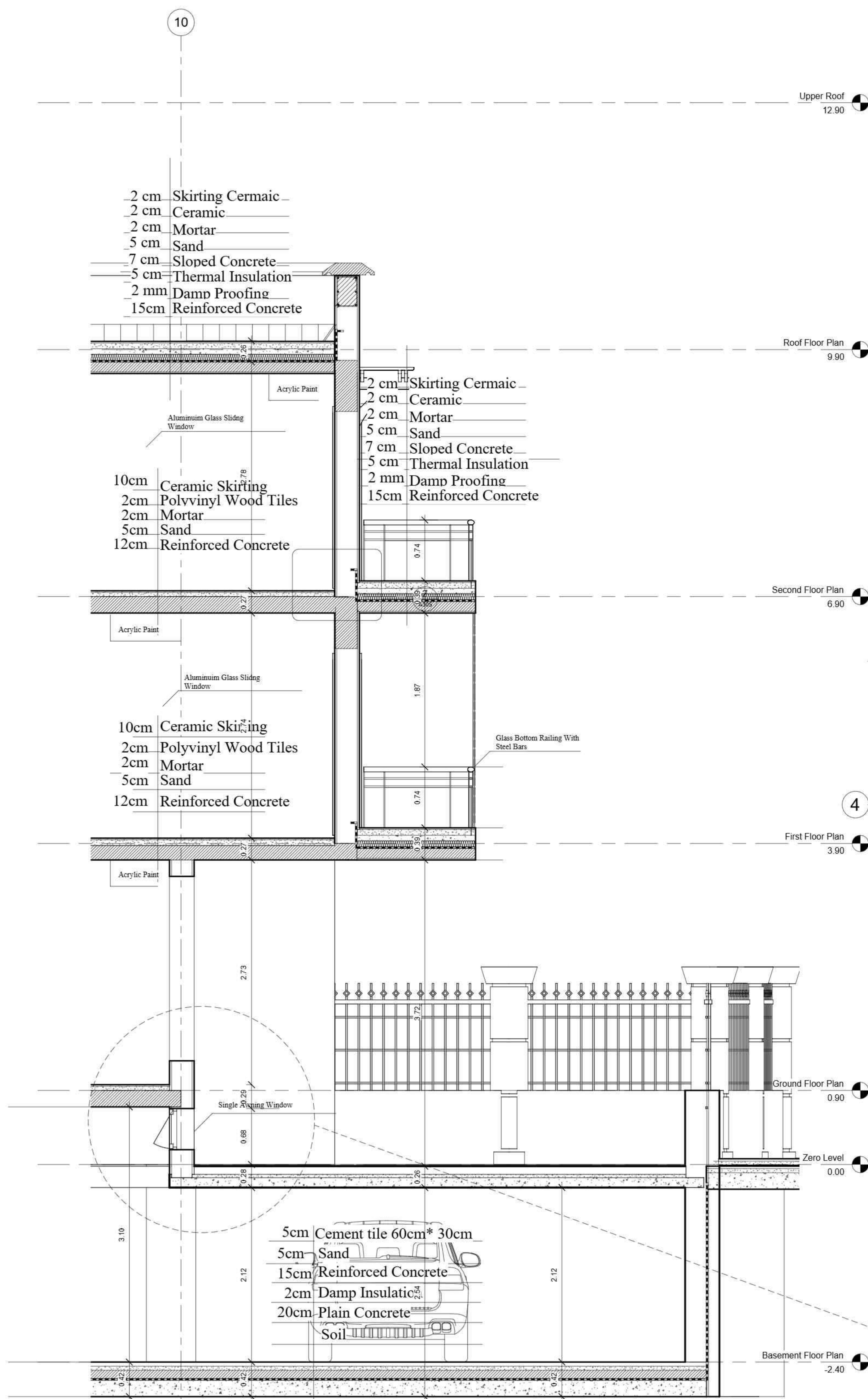
1 Wall Section 3 1 : 25
