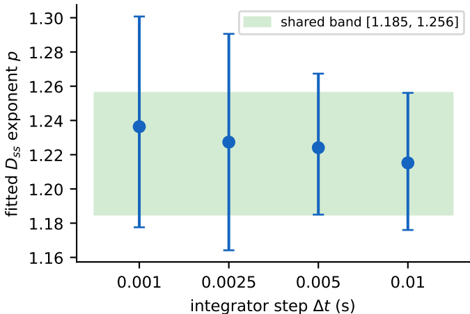
E10: numerics invariance over a 10\times \Delta t range
