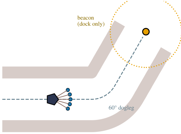
The Blind Harbor Transit (GNSS-denied dogleg)
