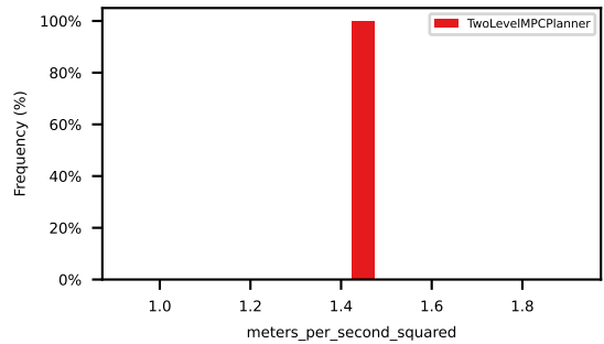
p90_ego_lon_acceleration
