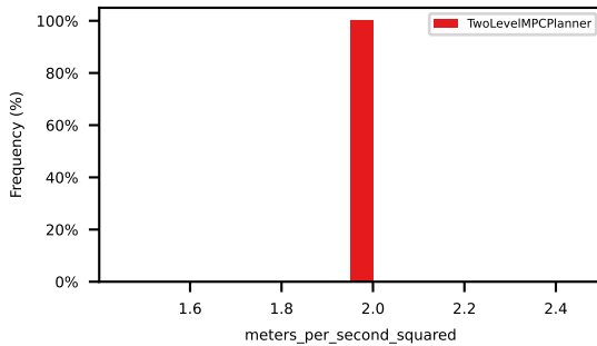
avg_ego_lon_acceleration
