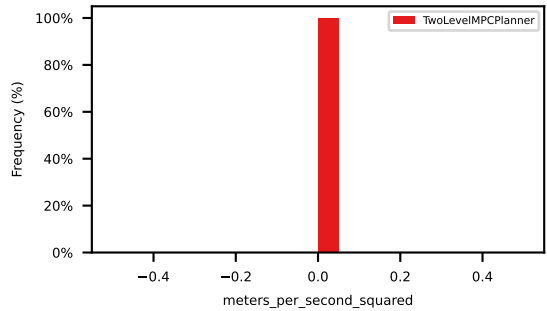
p90_ego_lat_acceleration
