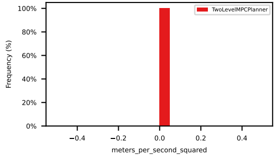
p90_ego_lat_acceleration
