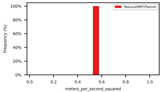
p90_ego_lon_acceleration
