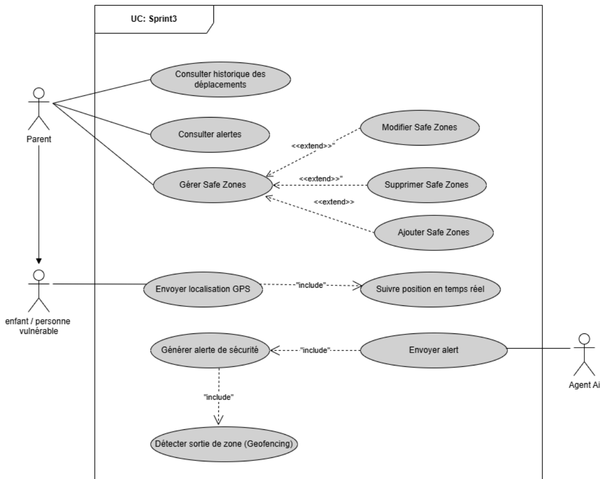
FIGURE 4.1 – Diagramme de cas d'utilisation – Sprint 3
