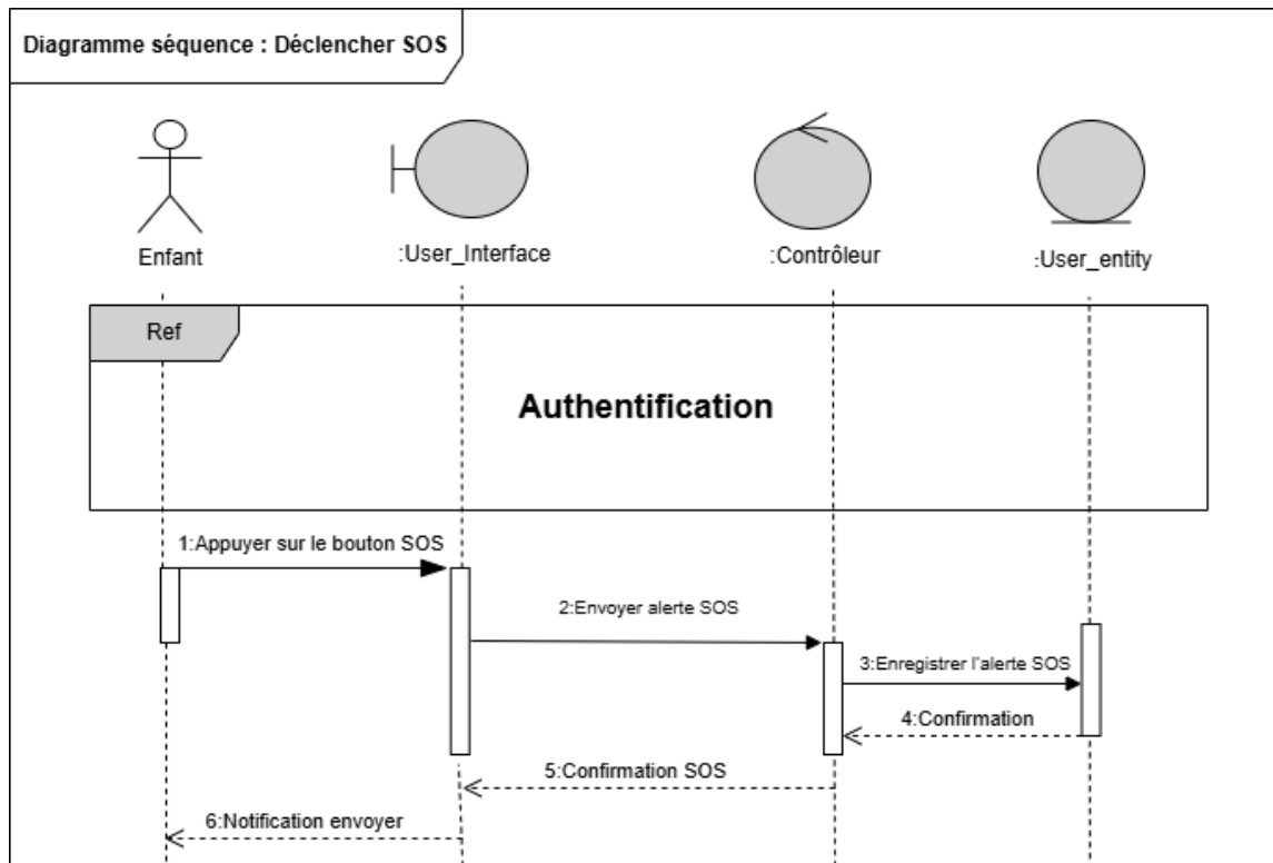
FIGURE 4.5 – Diagramme de séquence – Déclencher SOS
