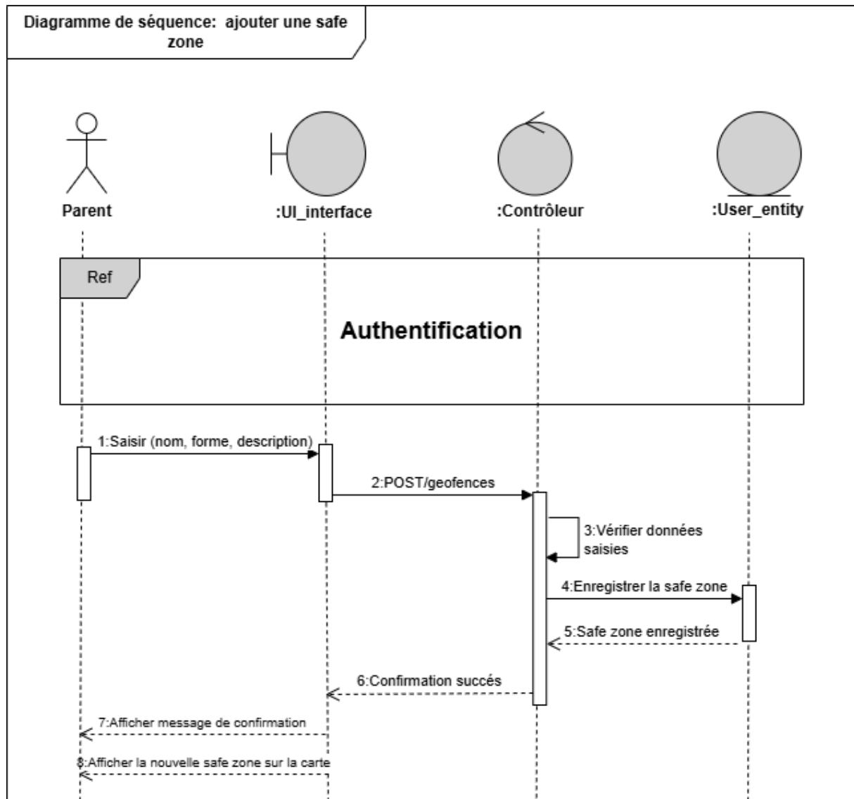
FIGURE 4.2 – Diagramme de séquence de Gestion des safezones
