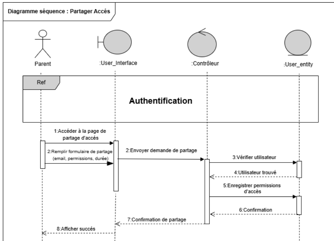
FIGURE 4.6 – Diagramme de séquence – Partager l'accès
