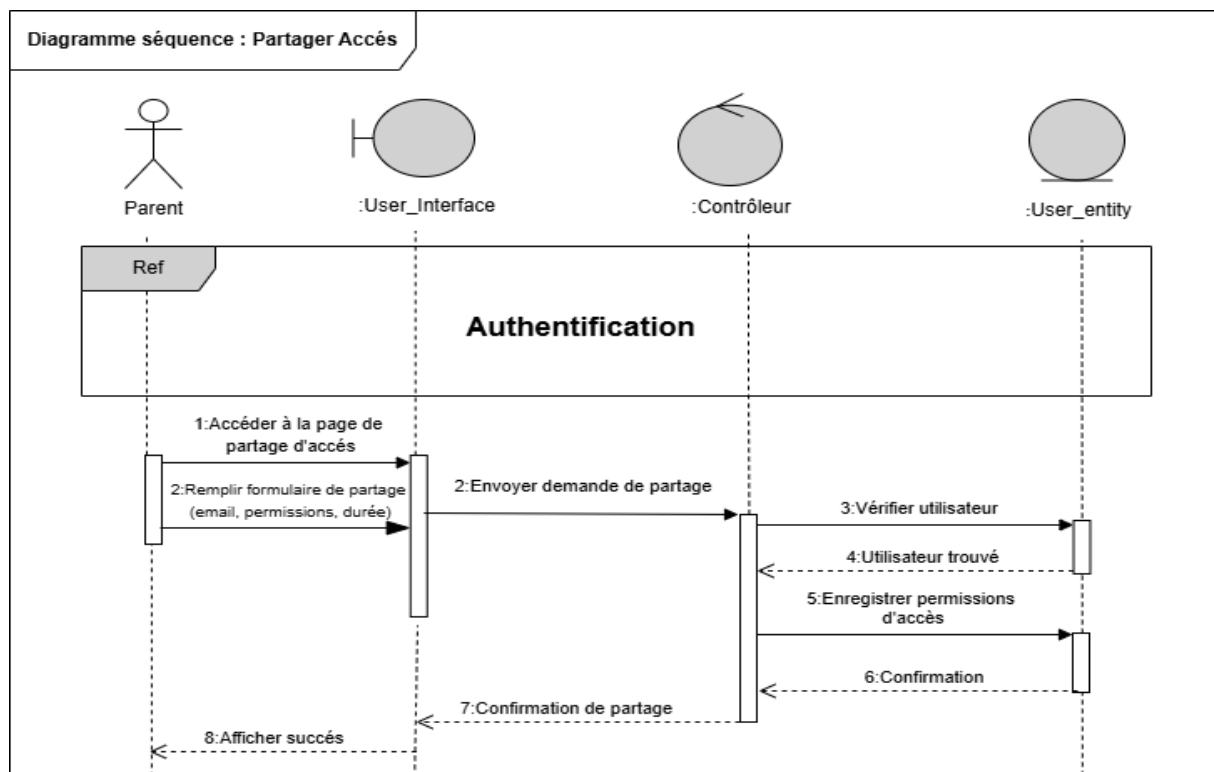
FIGURE 4.6 – Diagramme de séquence – Partager l'accès
