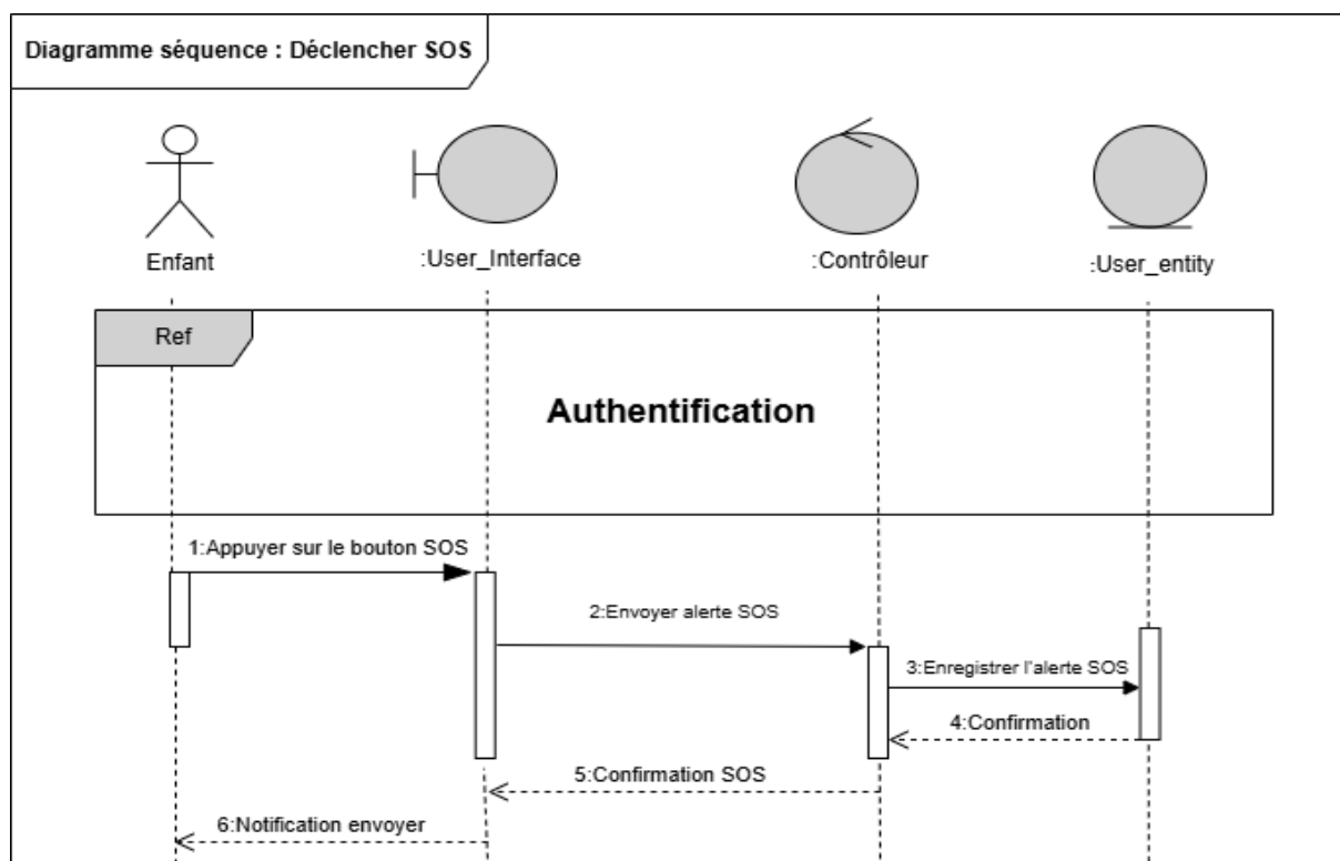
FIGURE 4.5 – Diagramme de séquence – Déclencher SOS
