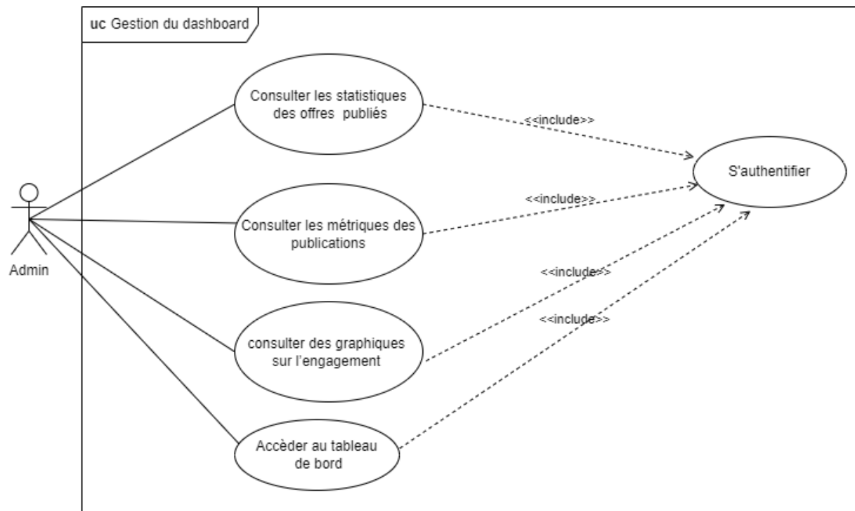
FIGURE 4.9 – Diagramme de cas d'utilisation de Gestion du dashboard
