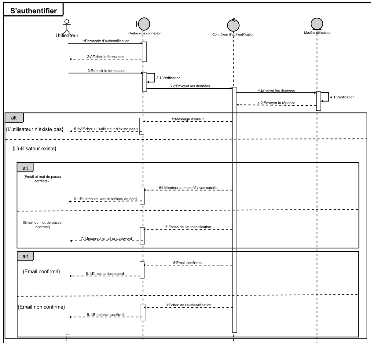
FIGURE 3.3 – Diagramme de séquence de S'authentifier (scénario classique)
