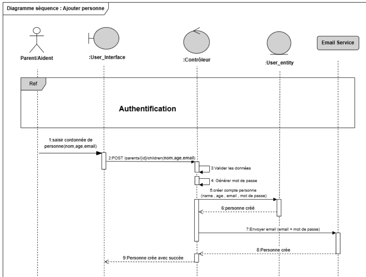
FIGURE 3.6 – Diagramme de séquence de Gestion des enfants
