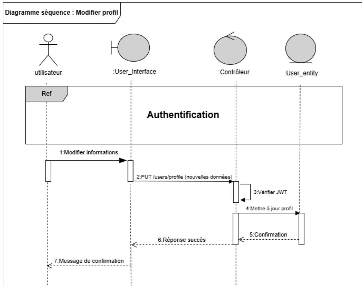
FIGURE 3.5 – Diagramme de séquence de Modifier profil
