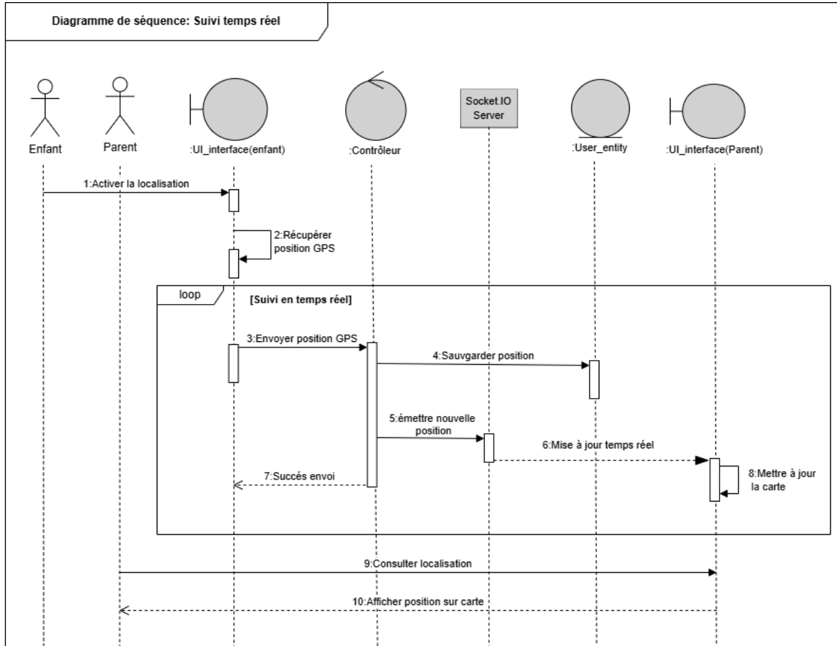
FIGURE 4.3 – Diagramme de séquence de Suivi en temps réel
