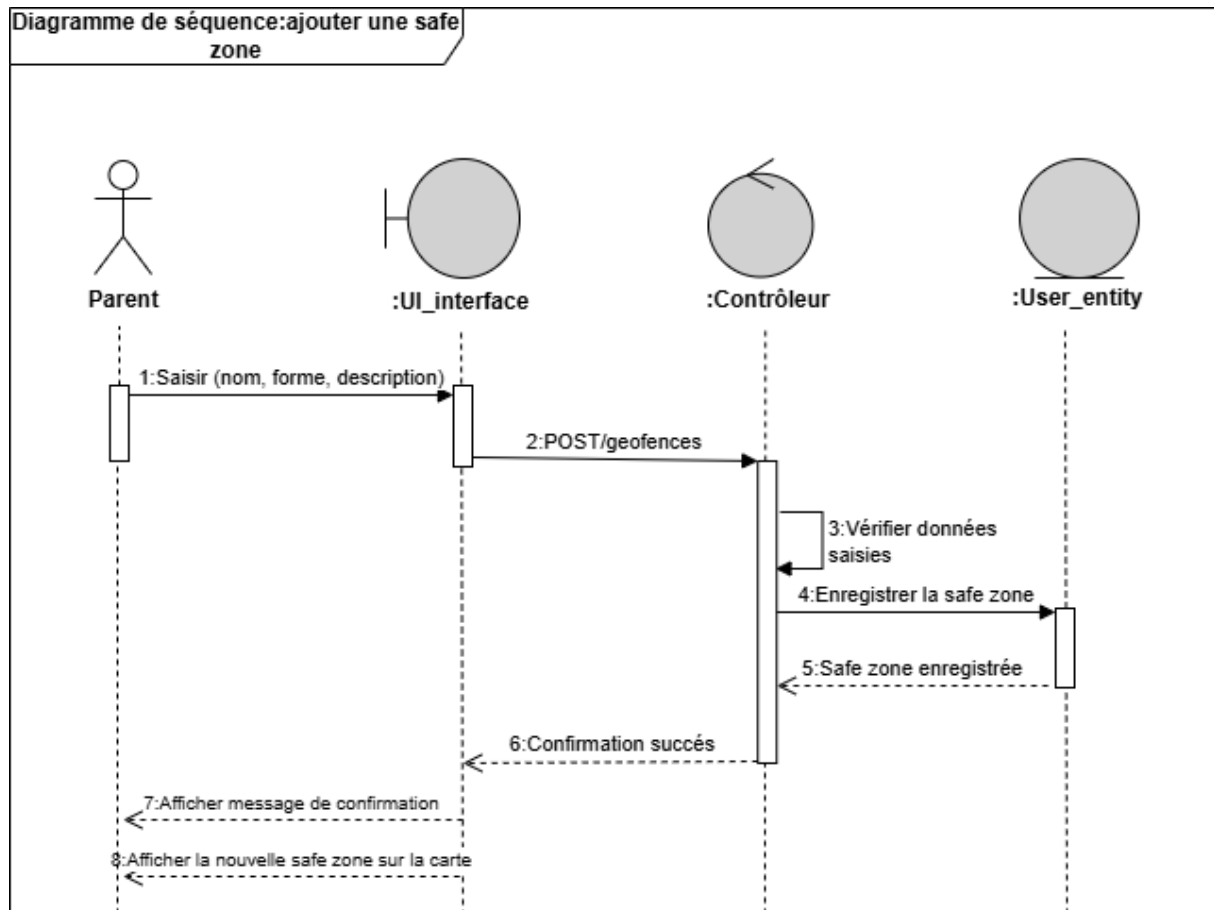
FIGURE 4.2 – Diagramme de séquence de Gestion des safezones
