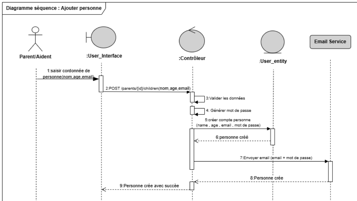
FIGURE 3.6 – Diagramme de séquence de Gestion des enfants
