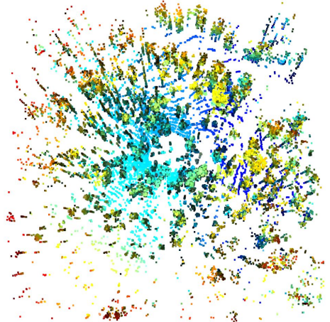
Logg3DNet & EgoNN
