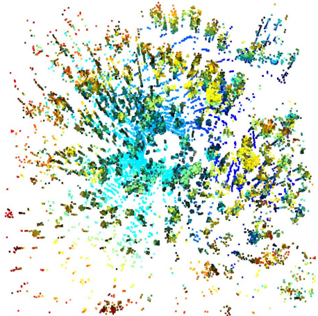
Logg3DNet & EgoNN
