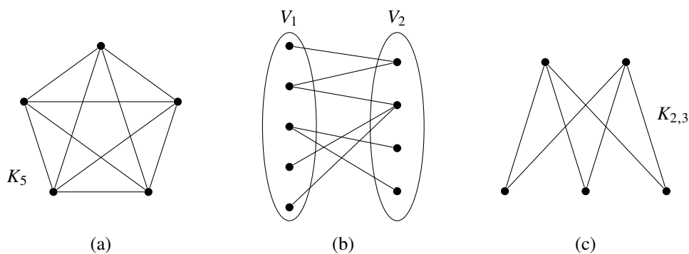
Figure A.1: (a) 完全图 (b) 二分图 (c) 完全二分图
