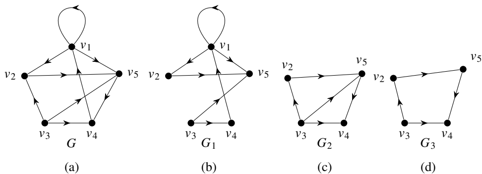
Figure A.2: G_1 是 G 的生成子图, G_2 是 G 的导出子图, G_3 是 G 的子图.
