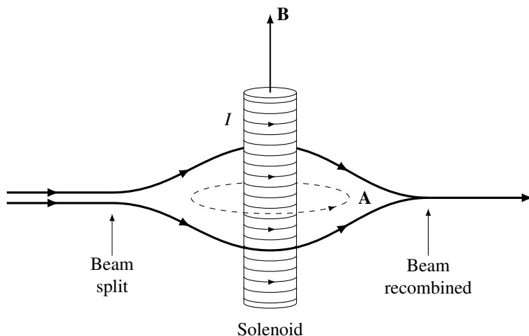
Figure D.2: Aharonov–Bohm 效应实验示意图
