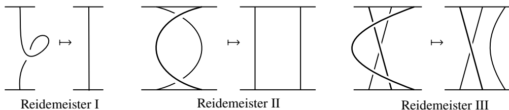
Figure 16.1: 三种 Reidemeister 变换, 反转辫的跨越方式亦是.
