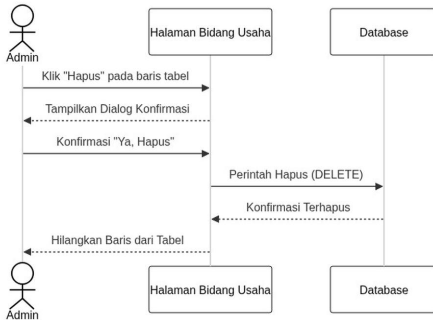
Gambar 3.12 Sequence Diagram Hapus Bidang Usaha
