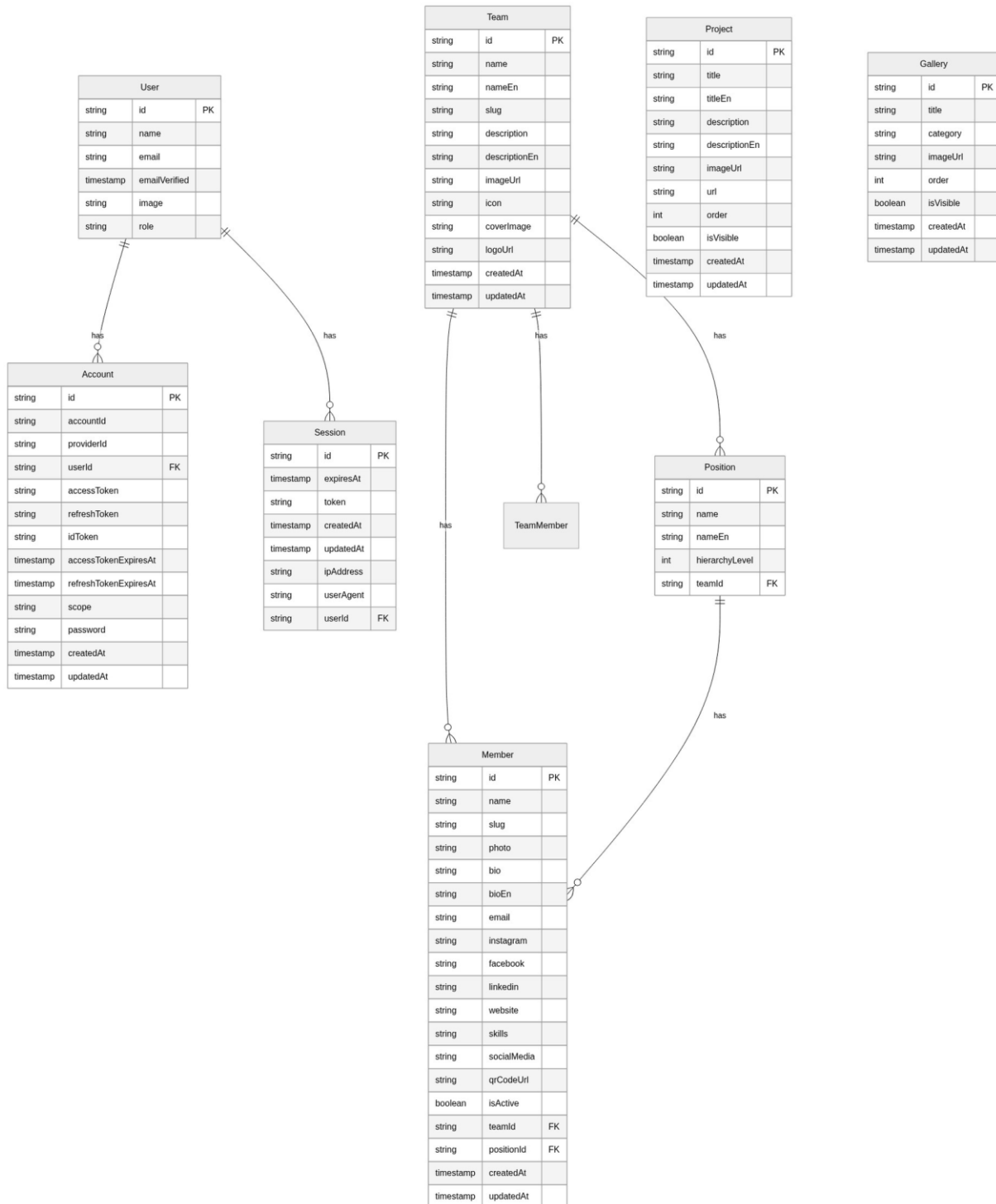
Gambar 3.19 Skema Relasi
