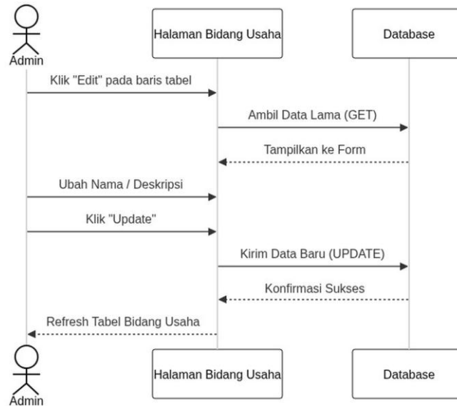
Gambar 3.11 Sequence Diagram Ubah (Edit) Bidang Usaha
