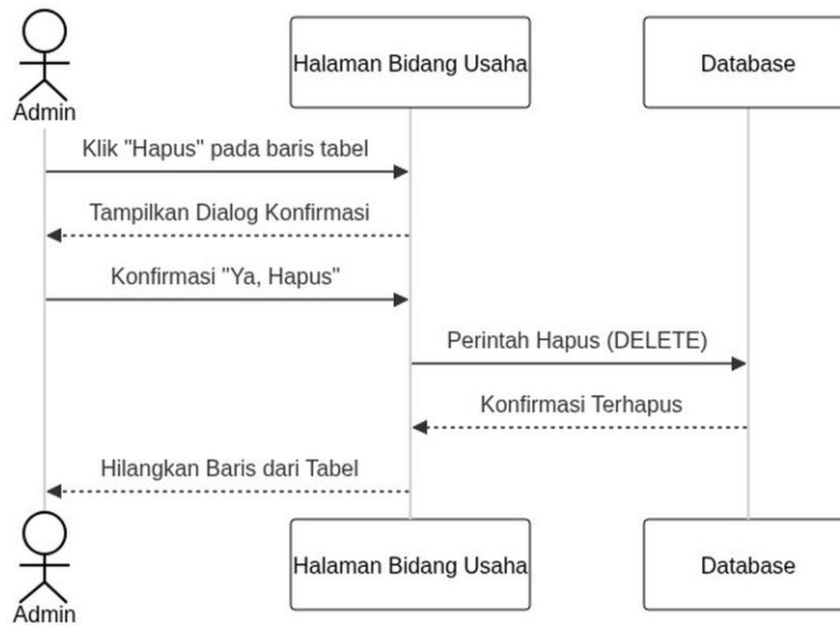
Gambar 3.12 Sequence Diagram Hapus Bidang Usaha
