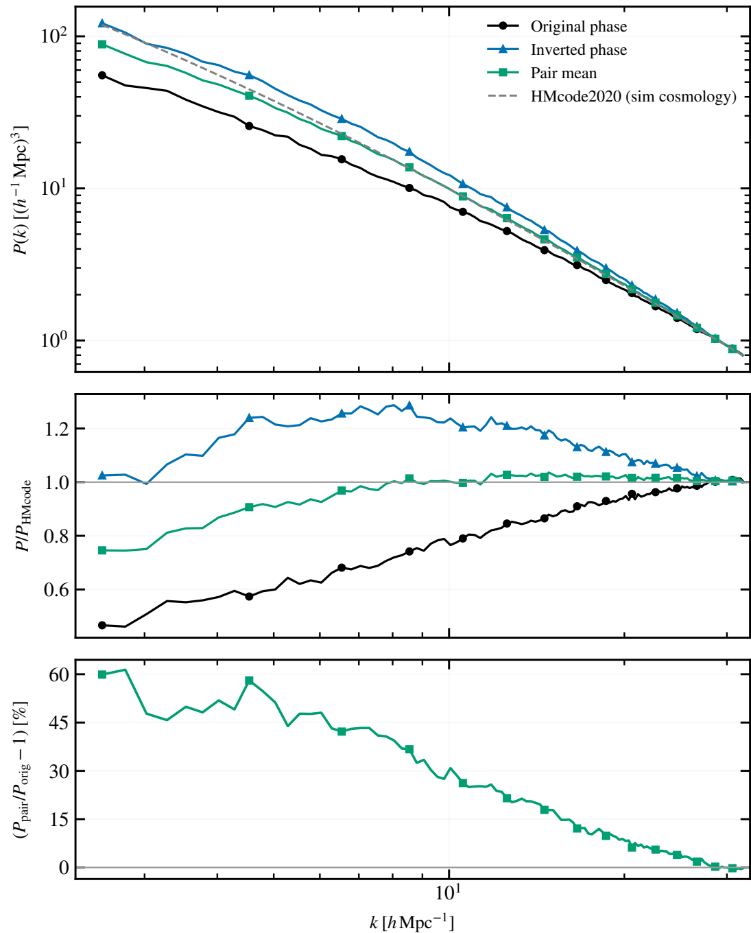
PL, z=0 , L=25\ h^{-1}\ \text{Mpc}
