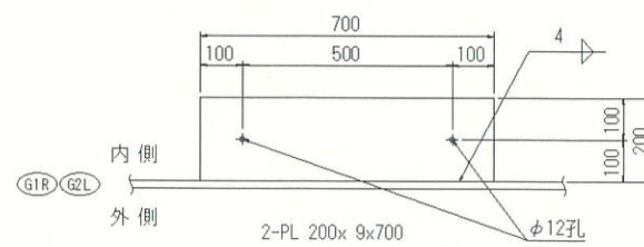
安定器箱固定板 S=1:10
