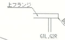
面取り処理図 S=1:10
