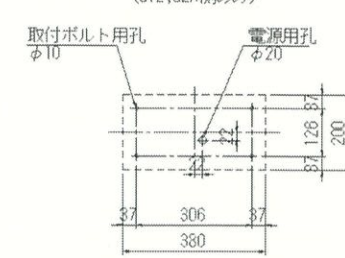
補助照明取付詳細 S=1:10
