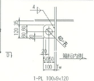
吊り金具詳細 S=1:10
