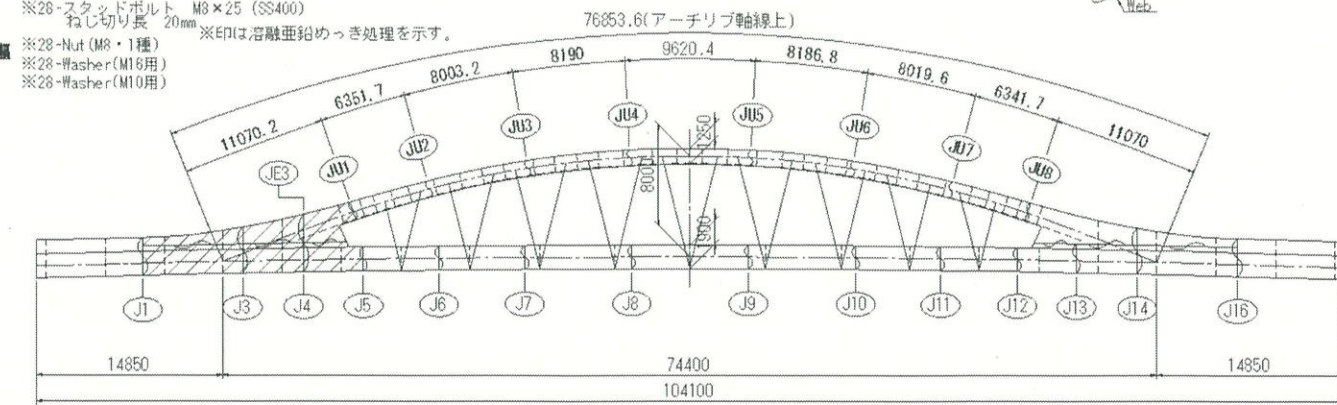
配置図 S=1:300
