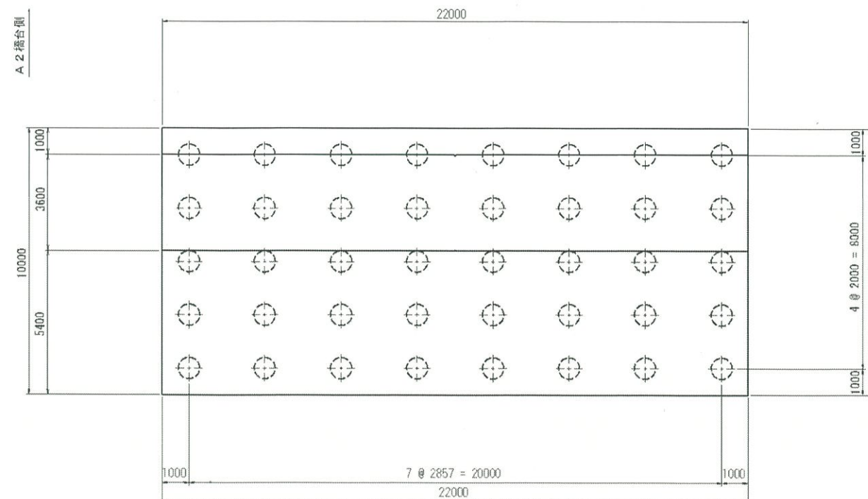
基礎平面図
