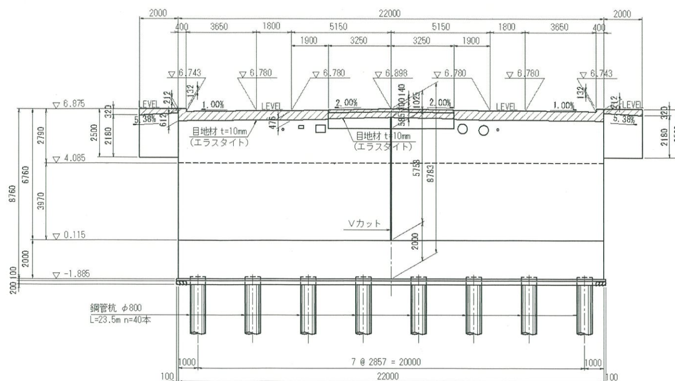
背面図
