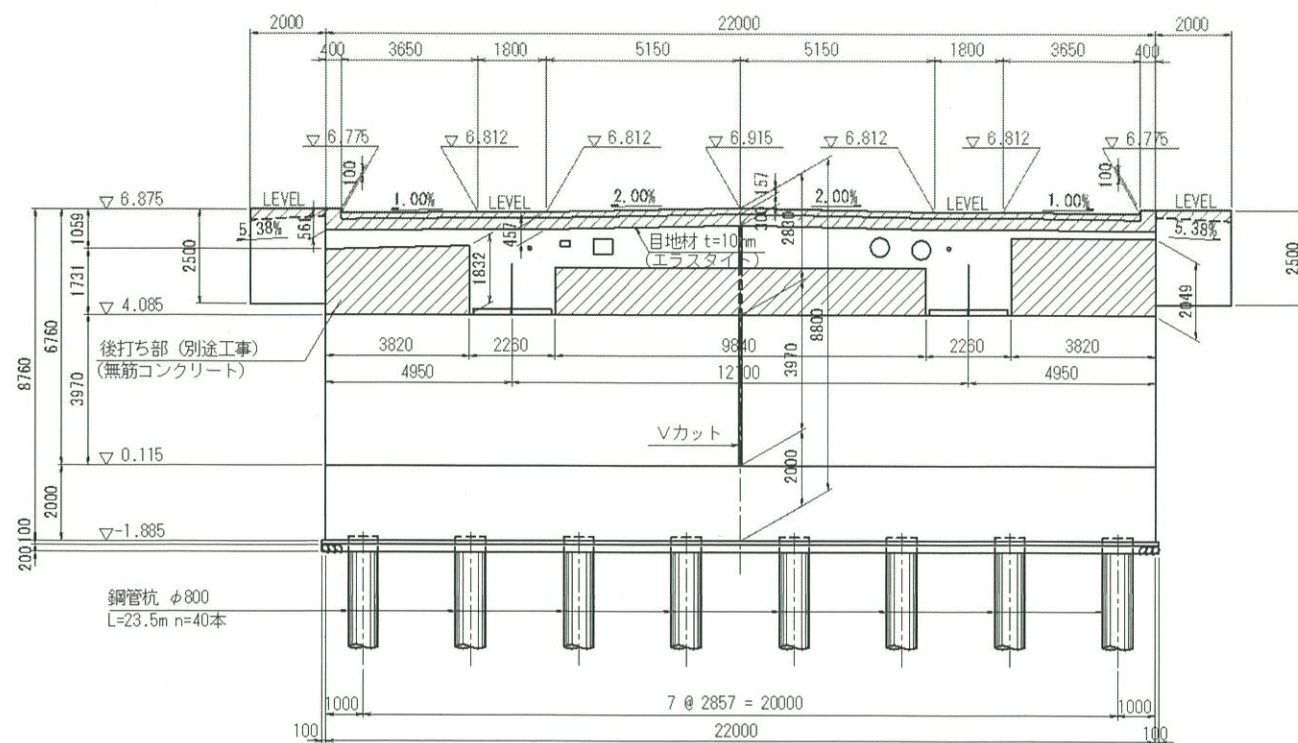
正面図
