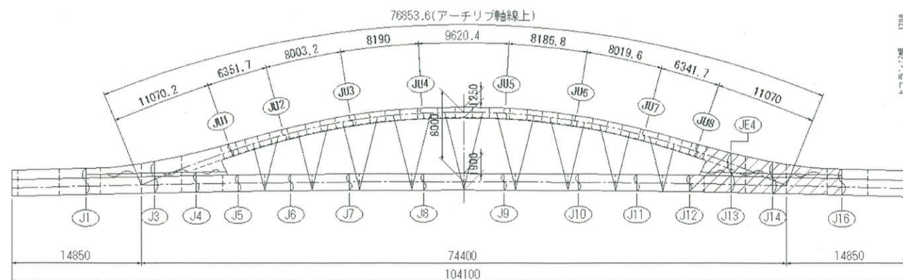
配置图 S=1:300
