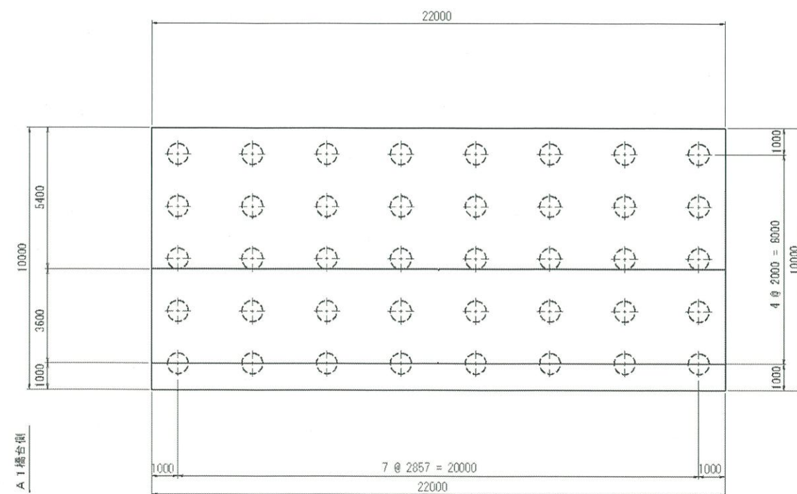
基礎平面図
