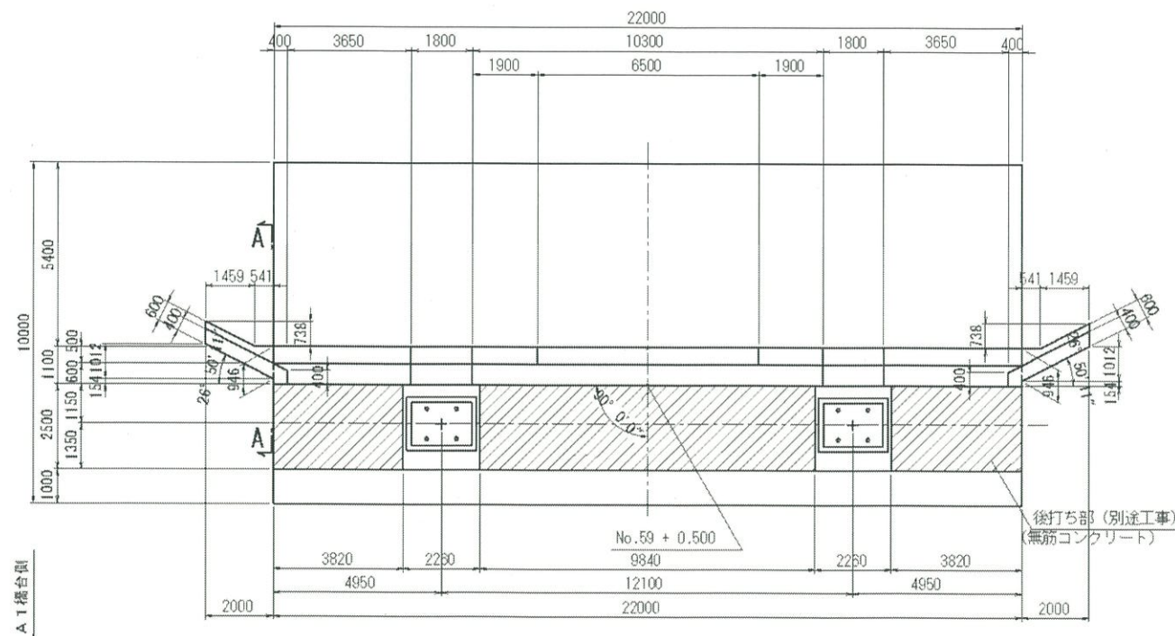
平面図
