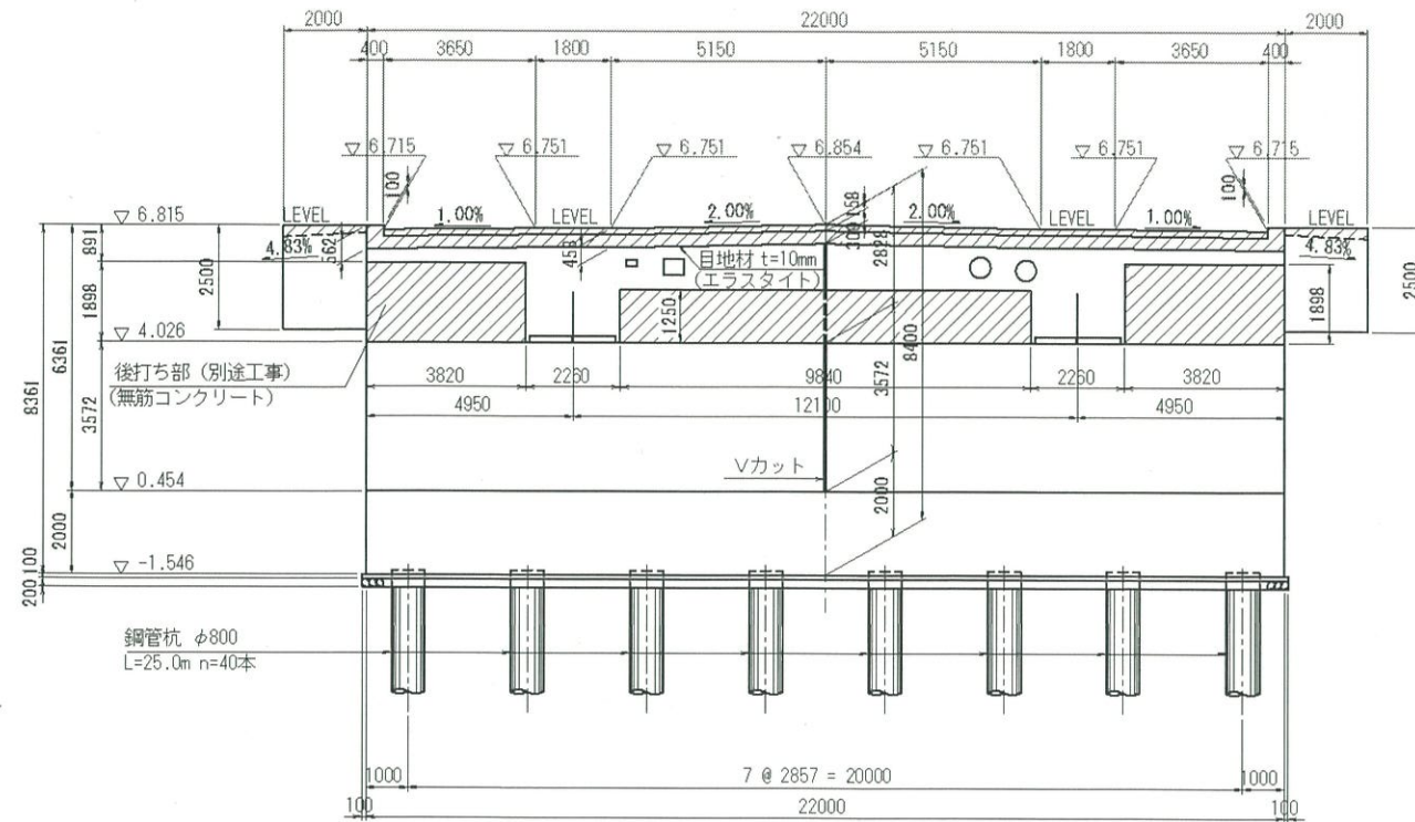
正面図
