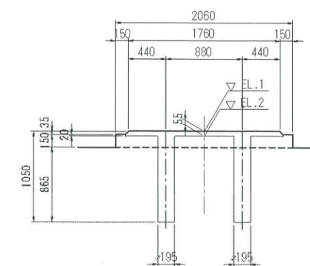
支承箱抜き詳細図 S=1:30
