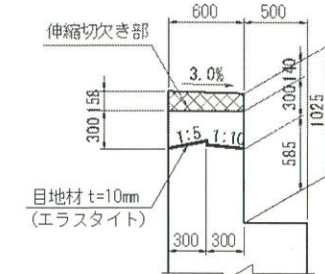
車道部
