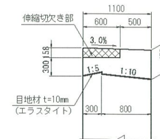
歩道部
