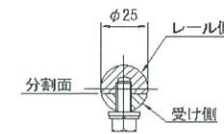
断面E-E S=1/2
