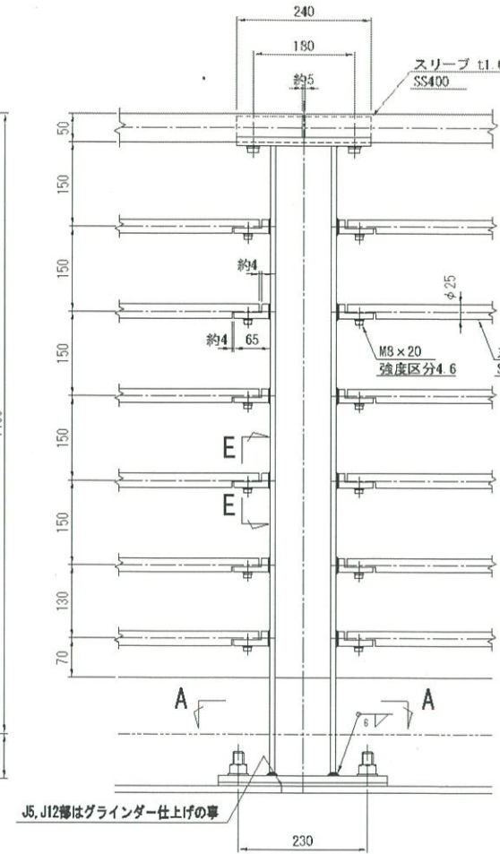
継手部
