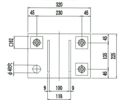
断面A-A
