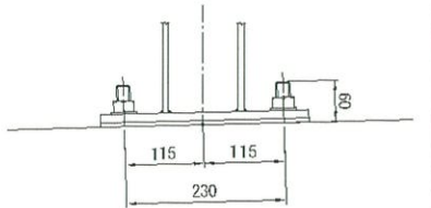
勾配部定着詳細図
