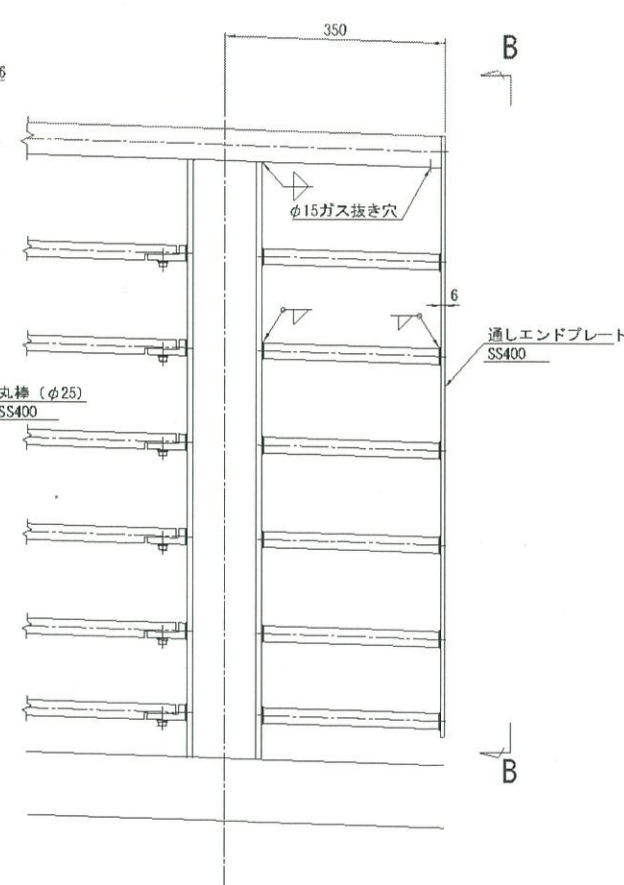
断面E-E S=1/2
