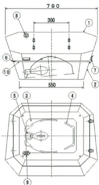
歩道灯 照明器具姿図 (橋脚部直付) カバー付 C (ランプ: HF80W)
