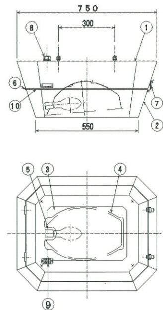
歩道灯 照明器具姿図 (橋脚部直付) カバー付 A (ランプ: HF80W)
