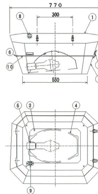
道路灯 照明器具姿図 (橋脚部直付) カバー付 B (ランプ: HF250W)
