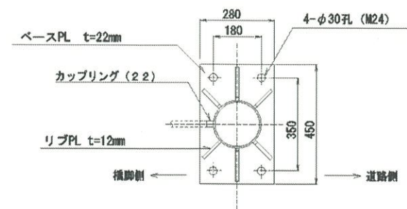
ベースプレート詳細図
