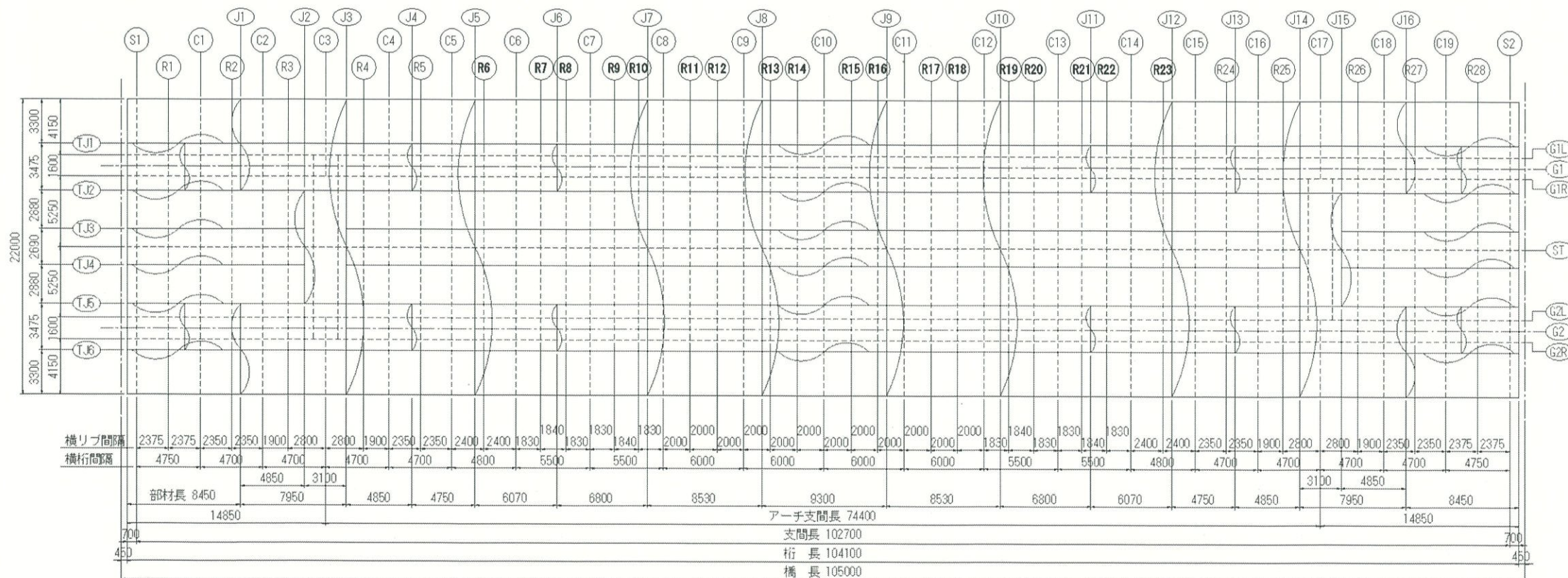
平面図
