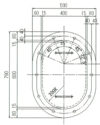
ジャッキ用マンホール詳細
