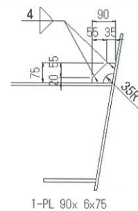
側板支持材詳細
