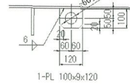
鋼床版用 吊金具詳細図
