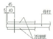
添接板端部詳細 S=1:5
