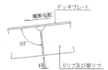
リブプレートの切断形状
