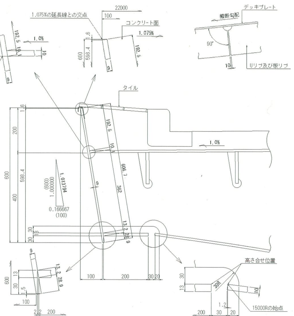
リブプレートの切断形状
