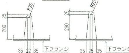
補剛桁部
