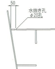
水抜き孔位置
