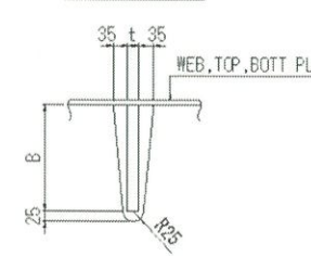
アーチリブ部
