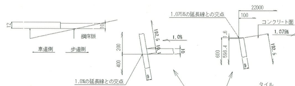
側縦桁部寸法詳細 S=1:5
