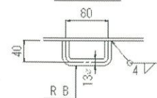
取手詳細
