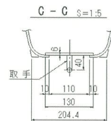
取手詳細
