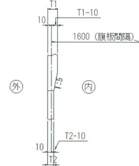
補剛桁ウェブ板厚変化詳細 S=1:5
