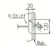
スカーラップ詳細図
