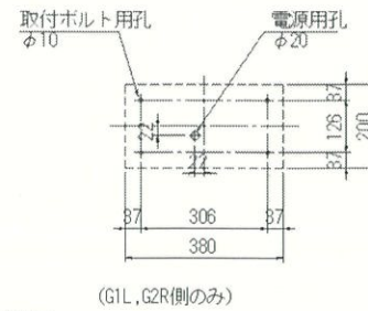
補助照明取付詳細 S=1:10
