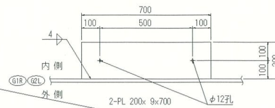
安定器箱固定板 S=1:10
