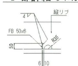
"B"部詳細 S=1:10
