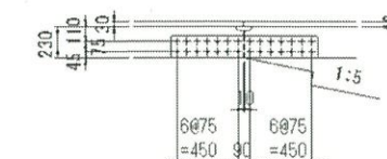
J1 上フランジ側縦リブ添接
