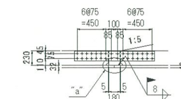
J1 下フランジ側縦リブ添接
