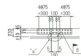
JE1 下フランジ側縦リブ添接
