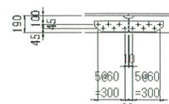
JE1 J1 水平補剛材添接
