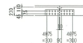
JE1 上フランジ側縦リブ添接
