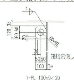
吊り金具詳細 S=1:10
