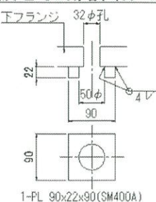
水抜き孔部詳細 S=1:5
