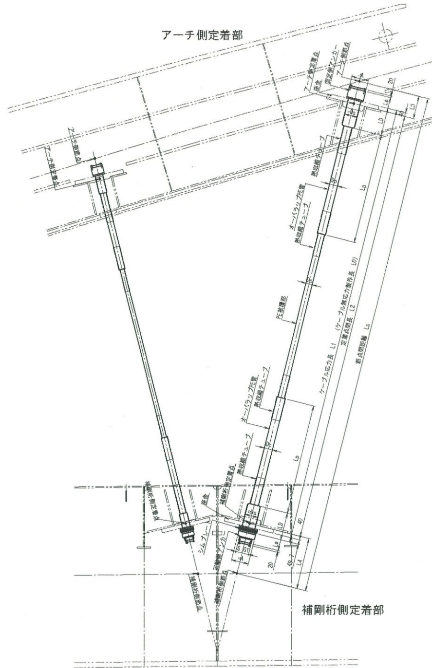
ケーブル図 S=1:20
