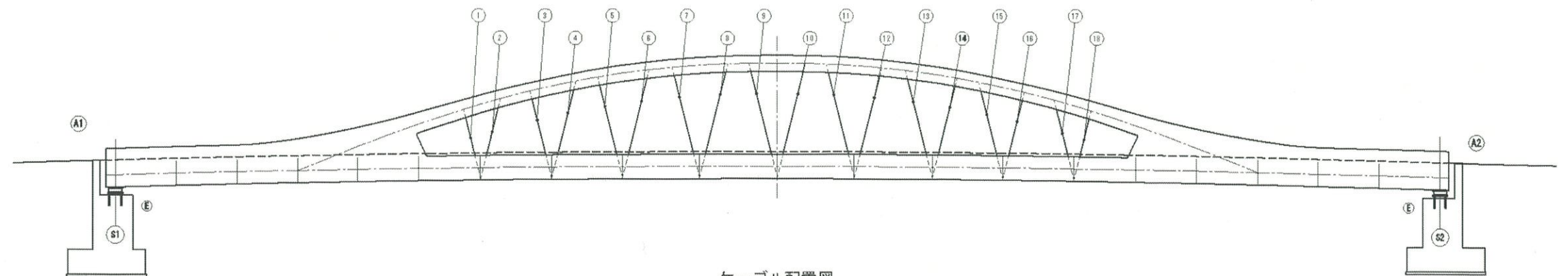
ケーブル配置図
