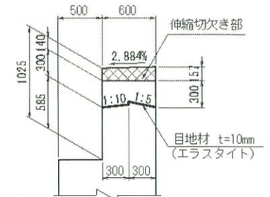
車道部
