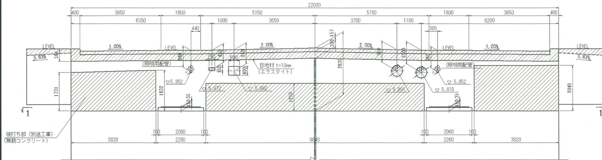
背面図
