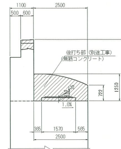
断面図
