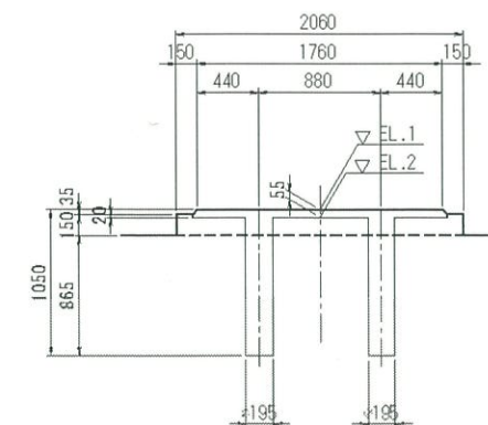
支承箱抜き詳細図 S=1:30
