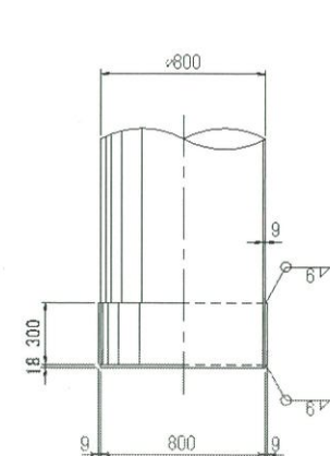
杭先端補強リング詳細図
