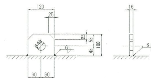
吊金具詳細図 S=1:5
