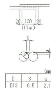
フレアー溶接詳細図
