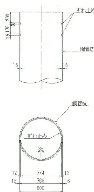
現場溶接ずれ止め詳細図
