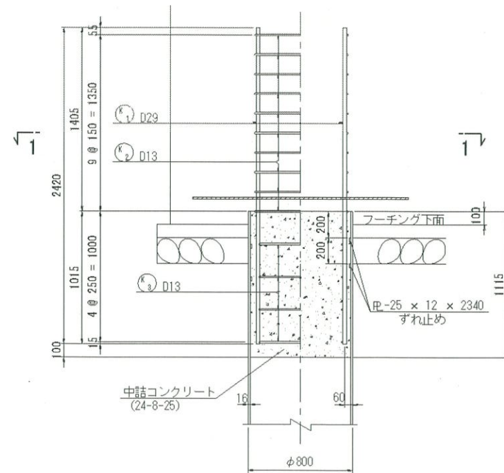
杭頭部詳細図
