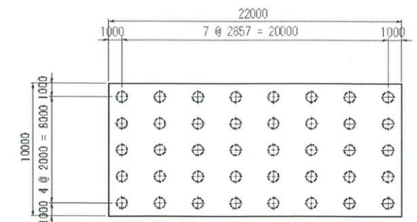
杭配置図
