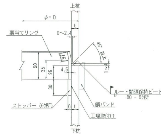
現場継手詳細図 S=1:2
