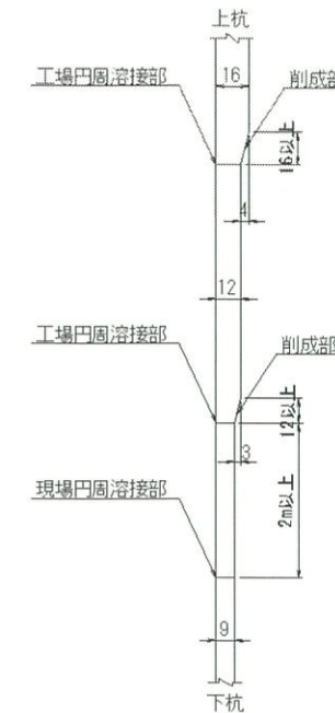
現場継手詳細図 S=1:2
