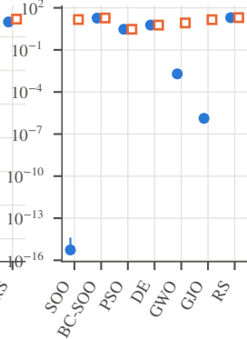
(d) ackley
