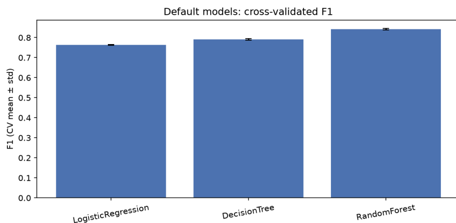
รูปที่ 9 ค่า F1 จาก Cross-Validation ของแบบจำลองทั้ง 3 ชนิด
