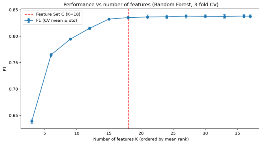
รูปที่ 8 ค่า F1 (Random Forest) เมื่อเพิ่มจำนวนตัวแปร (K) ตามลำดับความสำคัญ ใช้ประกอบการเลือก K = 18
