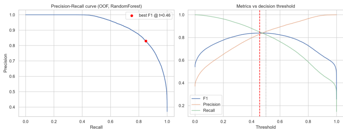
รูปที่ 11 เส้นโค้ง Precision-Recall และค่าตัวชี้วัดที่ Threshold ต่าง ๆ
